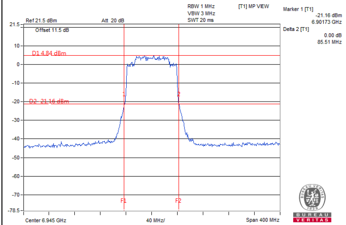
802.11ax (HE80) Full RU / Chain 0 : CH 199
