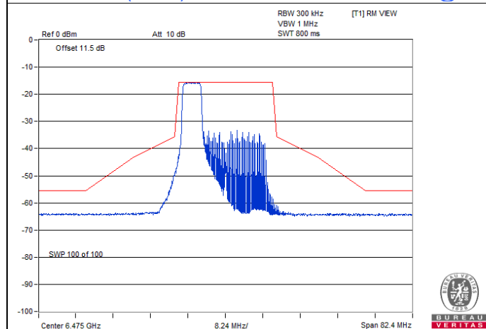
802.11ax (HE20) 52-tone RU / Chain 0 : CH 105@37
