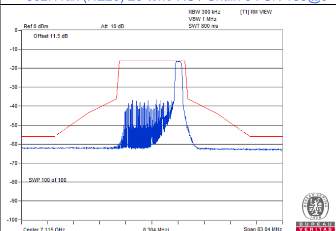
802.11ax (HE20) 26-tone RU / Chain 0 : CH 233@8
