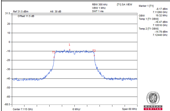
802.11ax (HE20) Full RU / Chain 0 : CH 233
