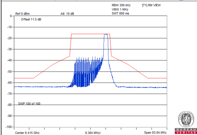
802.11ax (HE20) 26-tone RU / Chain 1 : CH 93@8
