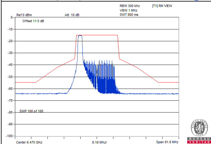
802.11ax (HE20) 26-tone RU / Chain 1 : CH 105@0
