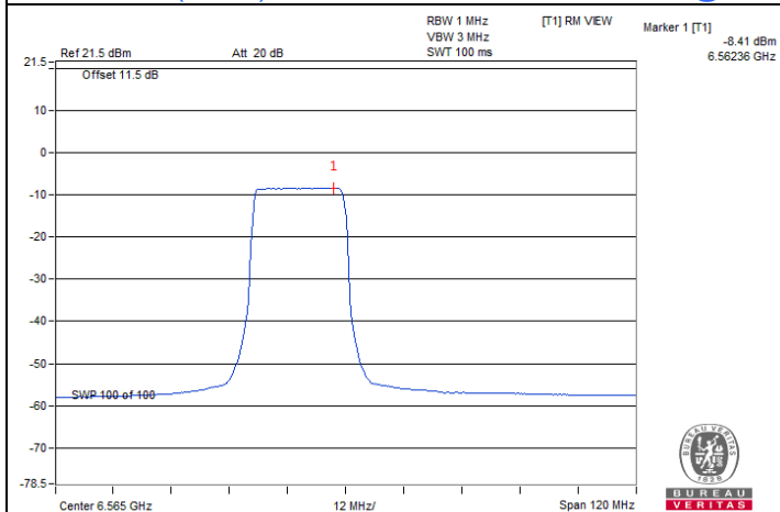
802.11ax (HE40) 242-tone RU / Chain 0 : CH 123@61
