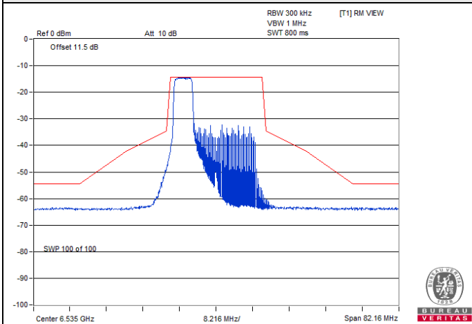
802.11ax (HE20) 52-tone RU / Chain 1 : CH 117@37
