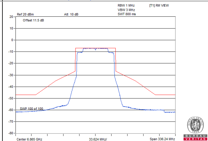
802.11ax (HE80) Full RU / Chain 1 : CH 183
