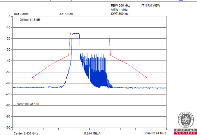
802.11ax (HE20) 52-tone RU / Chain 0 : CH 97@37
