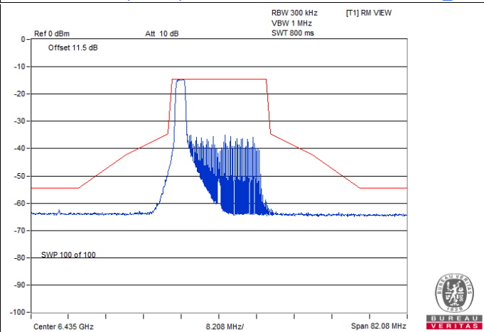
802.11ax (HE20) 26-tone RU / Chain 1 : CH 97@0
