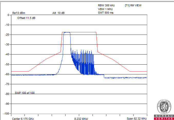
802.11ax (HE20) 52-tone RU / Chain 0 : CH 45@37
