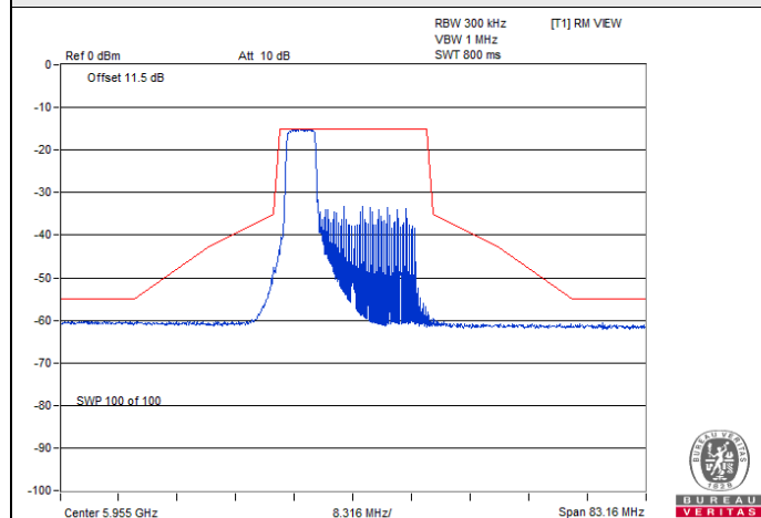
802.11ax (HE20) 52-tone RU / Chain 0 : CH 1@37
