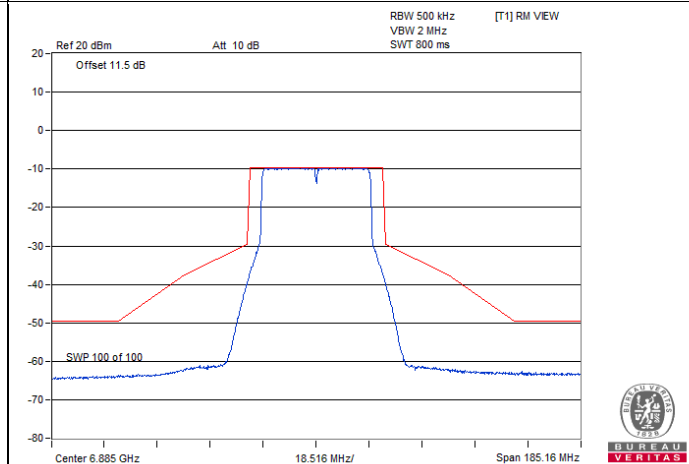
802.11ax (HE40) Full RU / Chain 1 : CH 187
