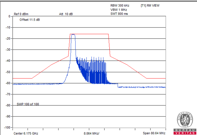
802.11ax (HE20) 26-tone RU / Chain 1 : CH 45@0
