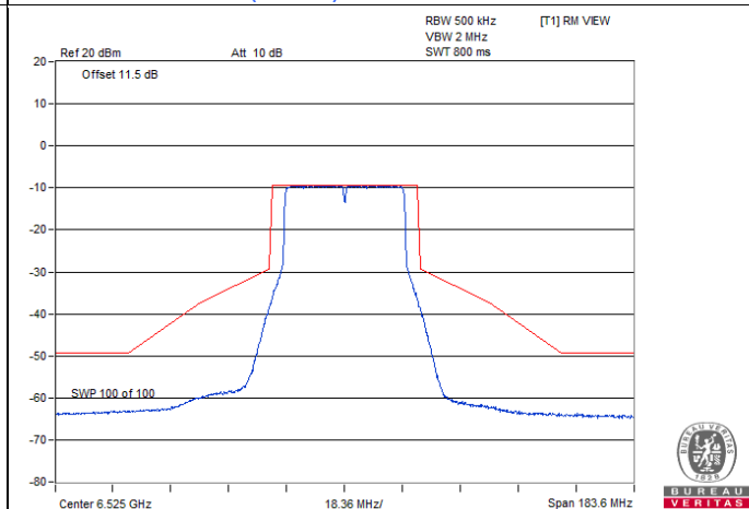
802.11ax (HE40) Full RU / Chain 0 : CH 115
