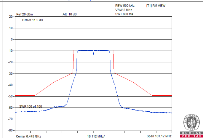
802.11ax (HE40) Full RU / Chain 0 : CH 99
