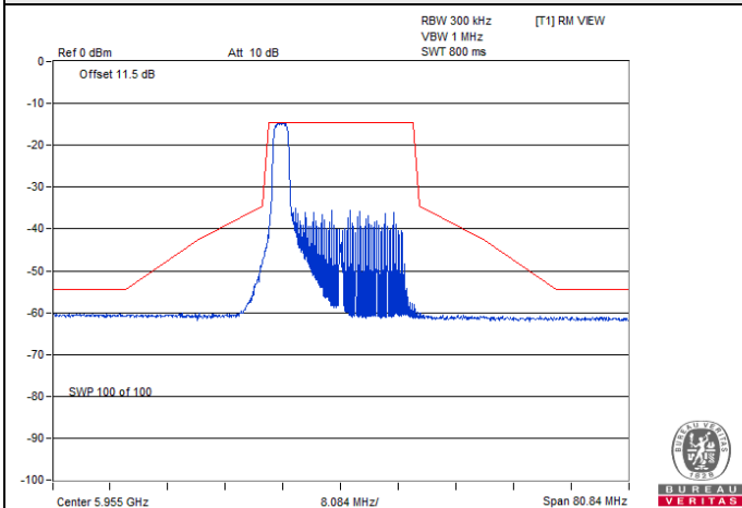
802.11ax (HE20) 26-tone RU / Chain 1 : CH 1@0
