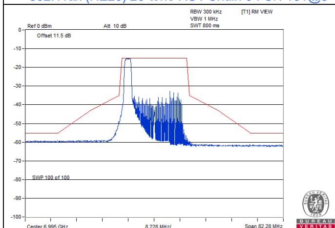
802.11ax (HE20) 26-tone RU / Chain 0 : CH 209@0
