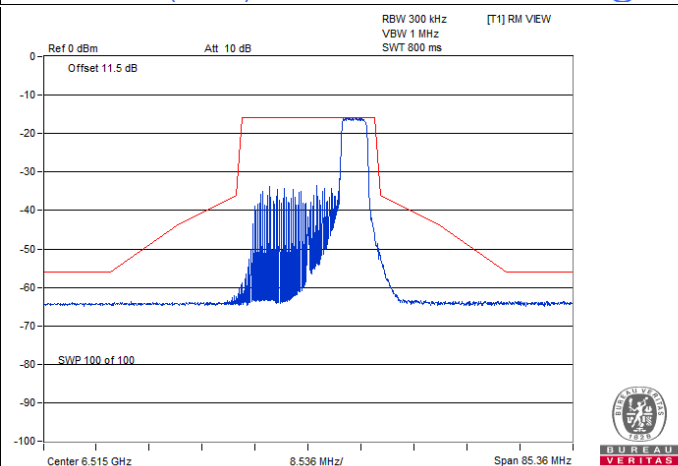
802.11ax (HE20) 52-tone RU / Chain 0 : CH 113@40
