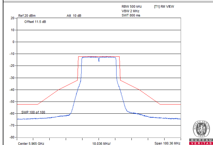
802.11ax (HE40) Full RU / Chain 0 : CH 3
