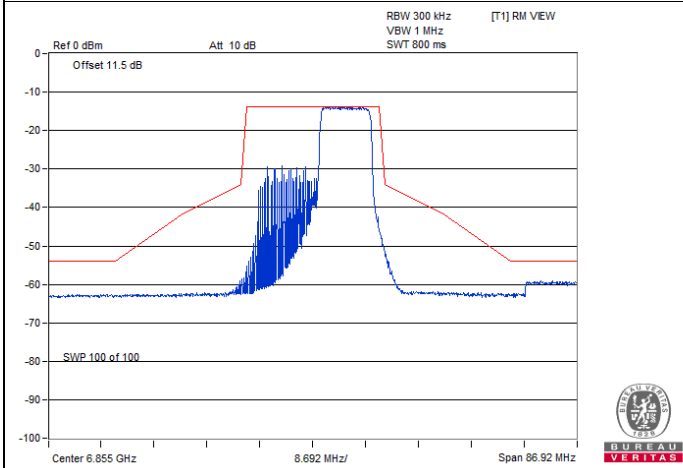
802.11ax (HE20) 106-tone RU / Chain 0 : CH 181@54
