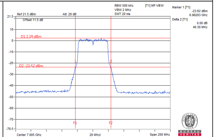
802.11ax (HE40) Full RU / Chain 0 : CH 211
