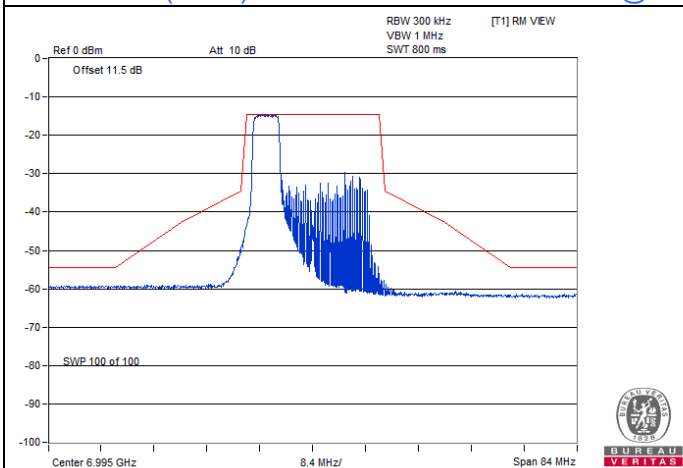
802.11ax (HE20) 52-tone RU / Chain 1 : CH 209@37
