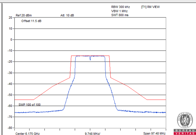
802.11ax (HE20) Full RU / Chain 0 : CH 45
