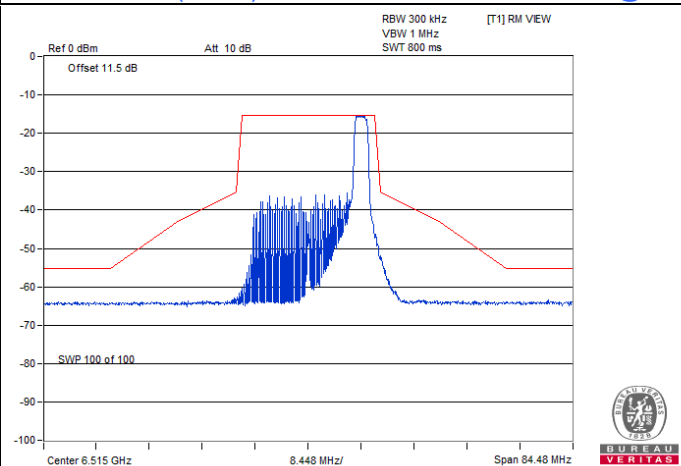
802.11ax (HE20) 26-tone RU / Chain 1 : CH 113@8
