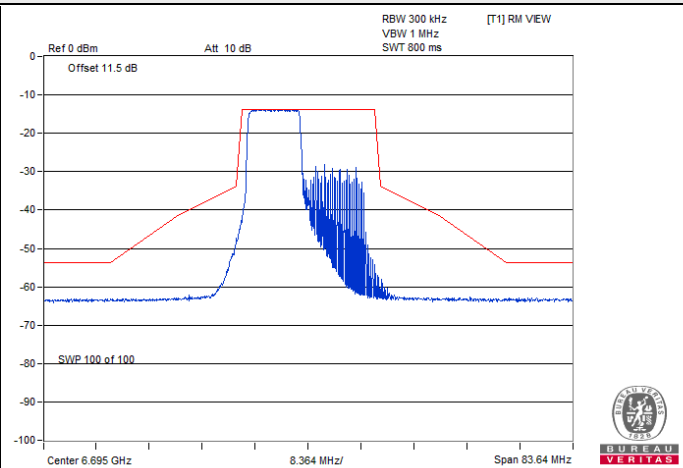
802.11ax (HE20) 106-tone RU / Chain 0 : CH 149@53
