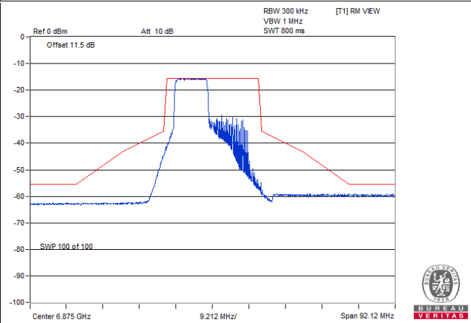
802.11ax (HE20) 106-tone RU / Chain 0 : CH 185@53
