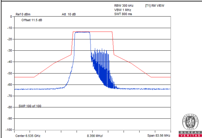
802.11ax (HE20) 106-tone RU / Chain 0 : CH 117@53
