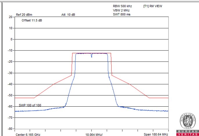
802.11ax (HE40) Full RU / Chain 0 : CH 43
