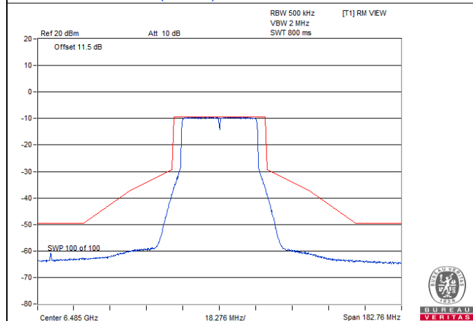
802.11ax (HE40) Full RU / Chain 0 : CH 107
