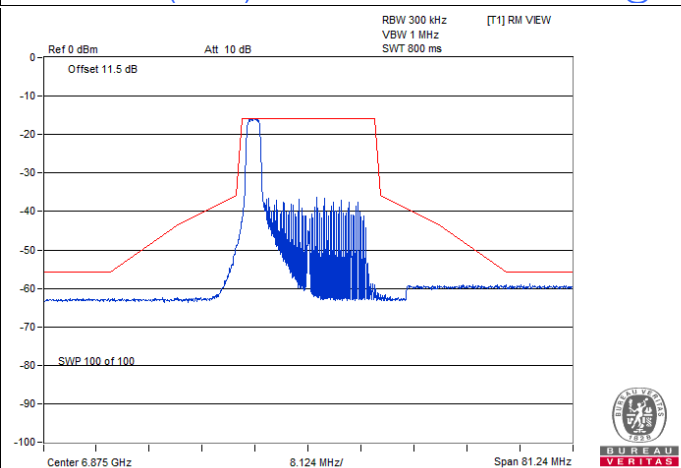
802.11ax (HE20) 26-tone RU / Chain 0 : CH 185@0
