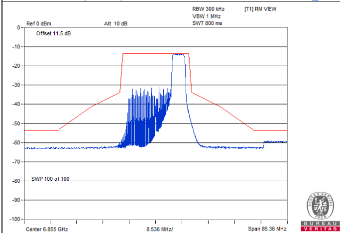
802.11ax (HE20) 52-tone RU / Chain 1 : CH 181@40
