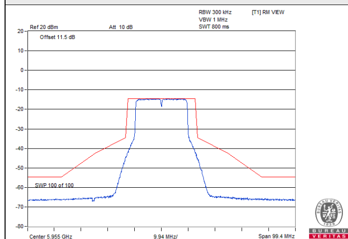
802.11ax (HE20) Full RU / Chain 0 : CH 1
