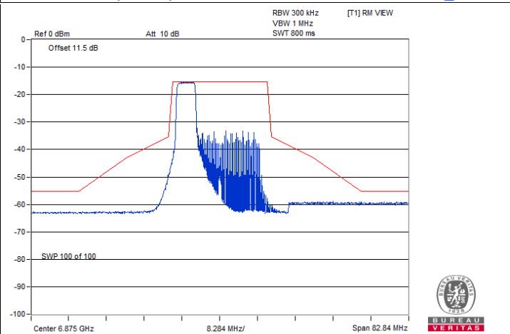
802.11ax (HE20) 52-tone RU / Chain 1 : CH 185@37
