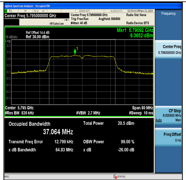
11N40MIMO-Ant7-5795
