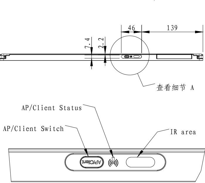
细节 A 比例 1.000
