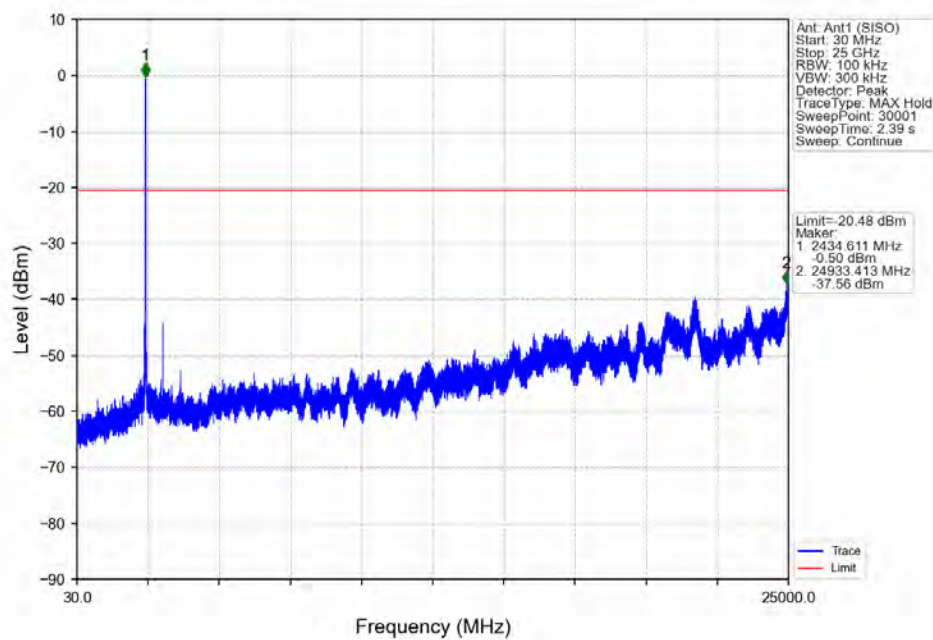
802.11ax(HEW40)_MCH_2437MHz_RU484_Left_Ant1 (SISO)_NTNV
