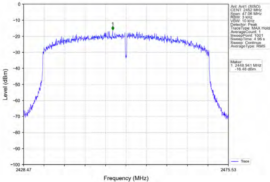
802.11ax(HEW40)_HCH_2452MHz_RU484_Left_Ant1 (SISO)_NTNV
