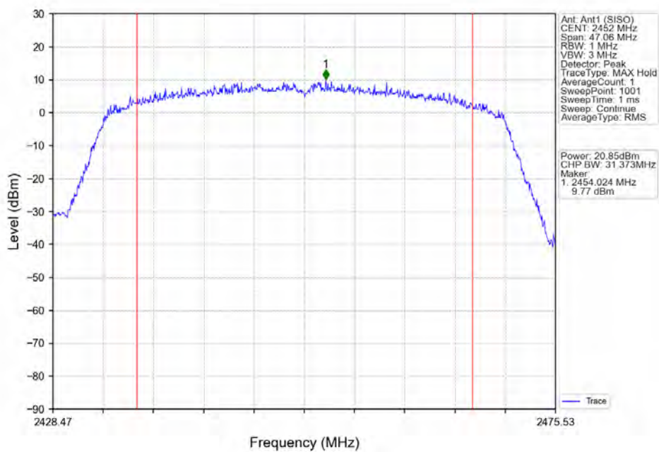
802.11ax(HEW40)_HCH_2452MHz_RU484_Left_Ant1 (SISO)_NTNV
