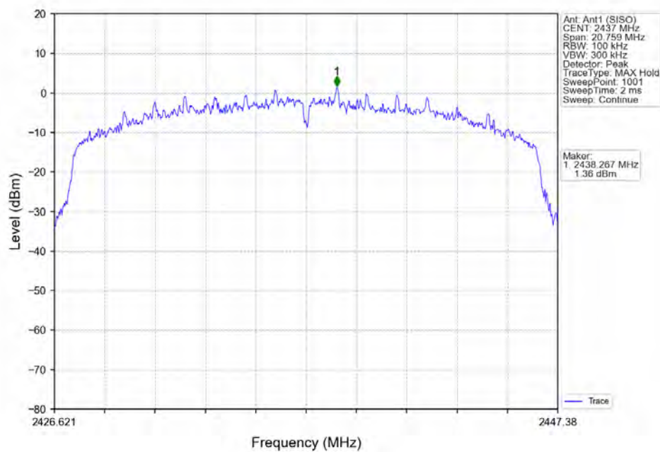
802.11ax(HEW20)_MCH_2437MHz_RU242_Left_Ant1 (SISO)_NTNV
