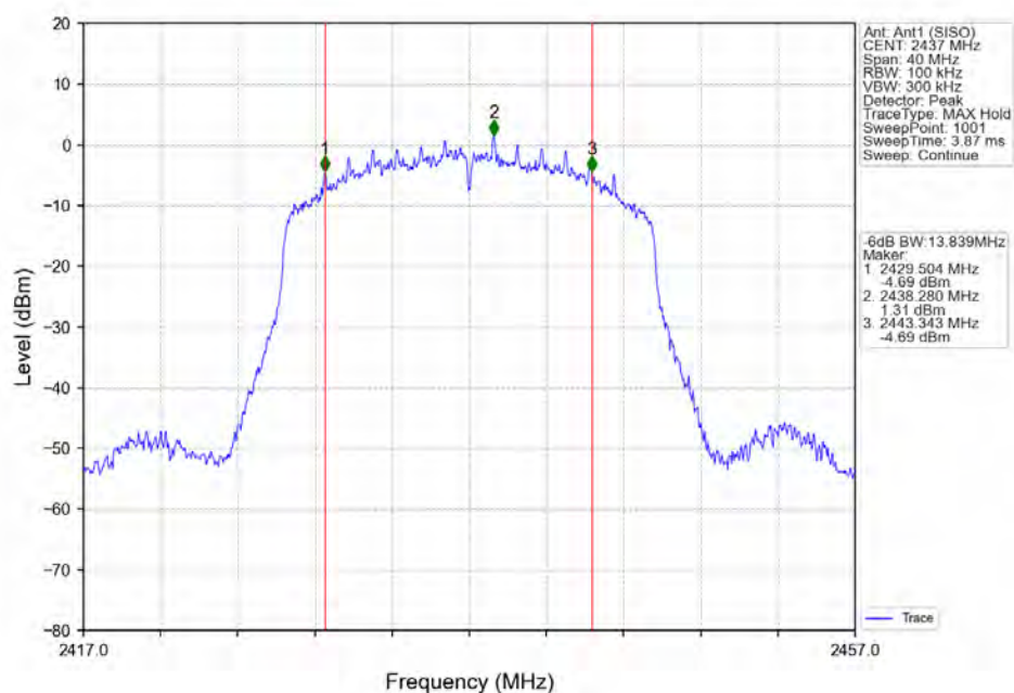
802.11ax(HEW20)_MCH_2437MHz_RU242_Left_Ant1 (SISO)_NTNV
