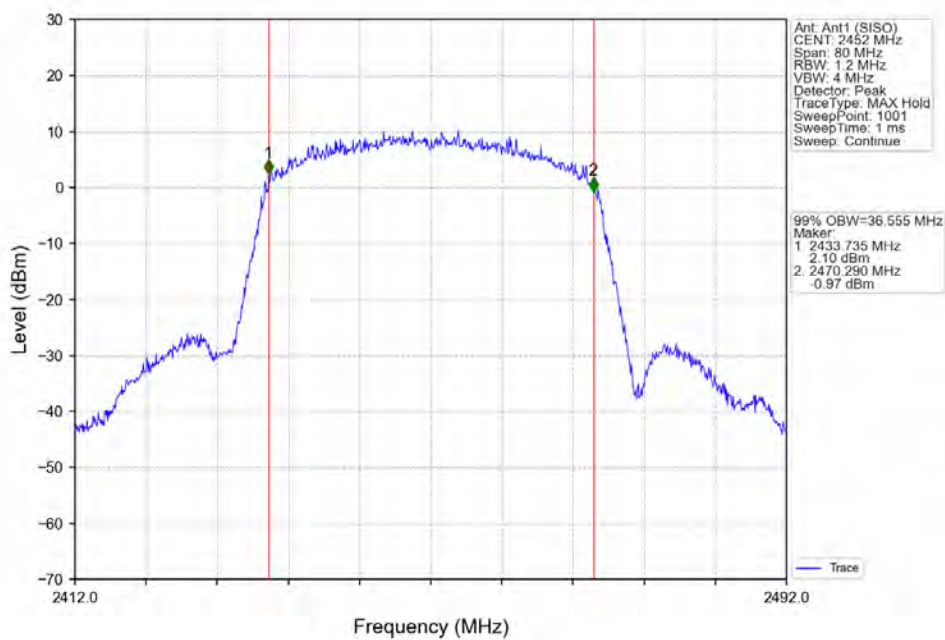
802.11ax(HEW40)_HCH_2452MHz_RU484_Left_Ant1 (SISO)_NTNV
