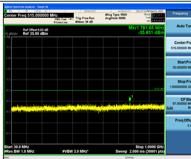
Band41-10MHz-QPSK-41540-1RB#0-Range4:1000~5000MHz
