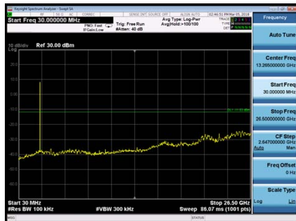
DH5 -CH78 0.03GHz to 26.5GHz
