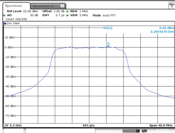
802.11a_5200
