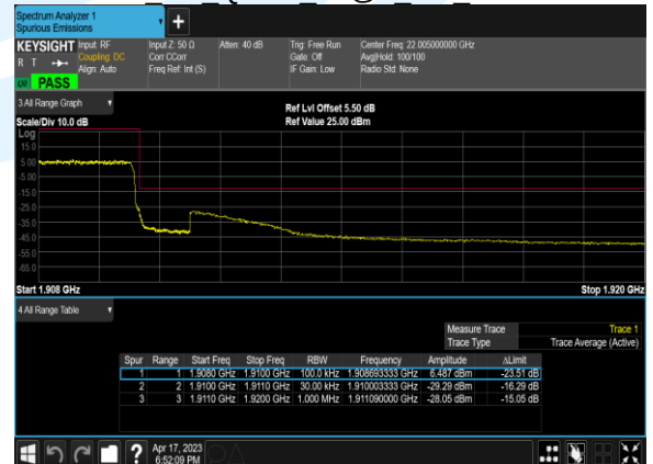
B2 3M QPSK 15@0 CH 19185
