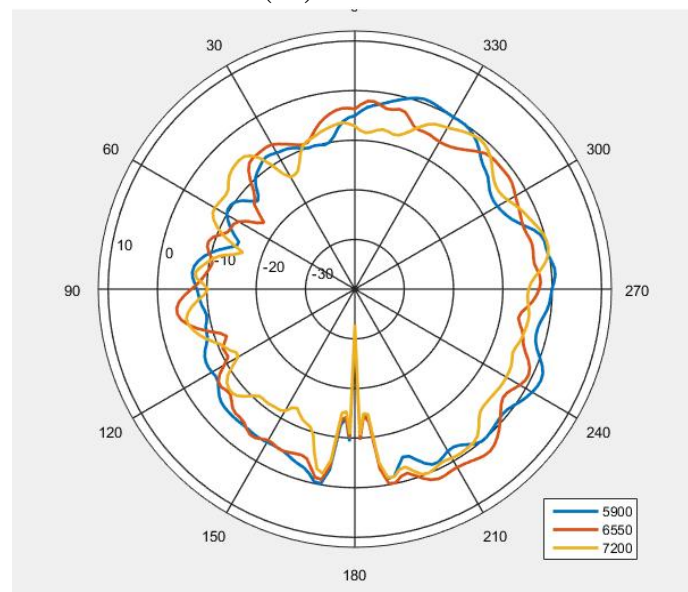
Y0Z(E2) 5925-7125MHz
