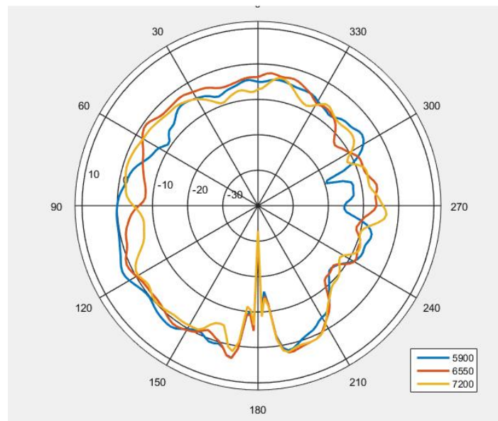
Y0Z(E2) 5925-7125MHz
