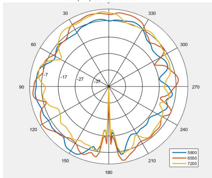
Y0Z(E2) 5925-7125MHz
