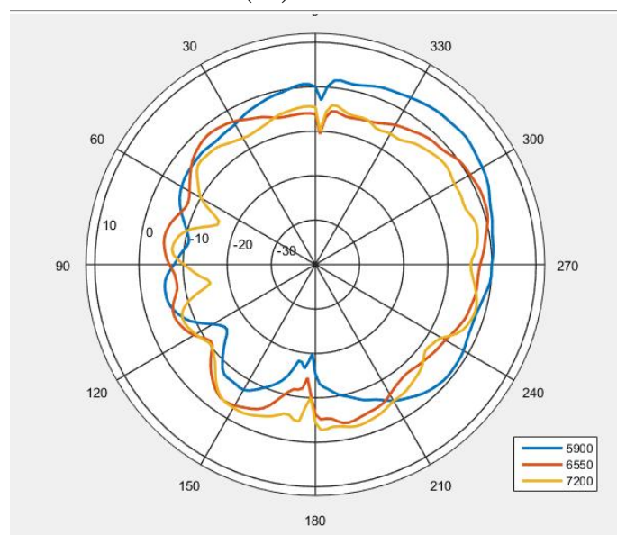
Y0Z(E2) 5925-7125MHz
