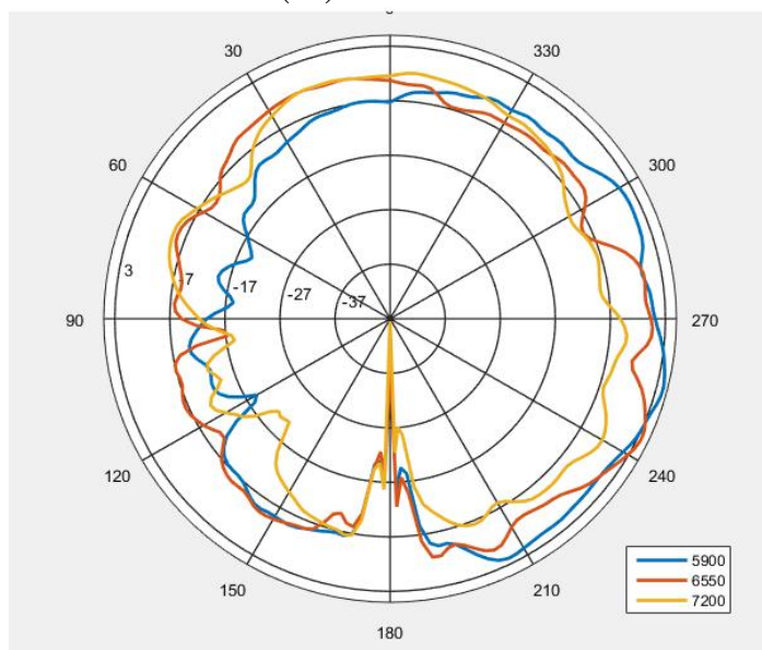
Y0Z(E2) 5925-7125MHz
