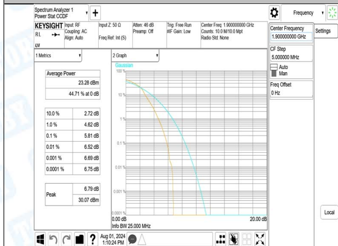
Band2-20MHz-16QAM-19100-1RB#0-PASS
