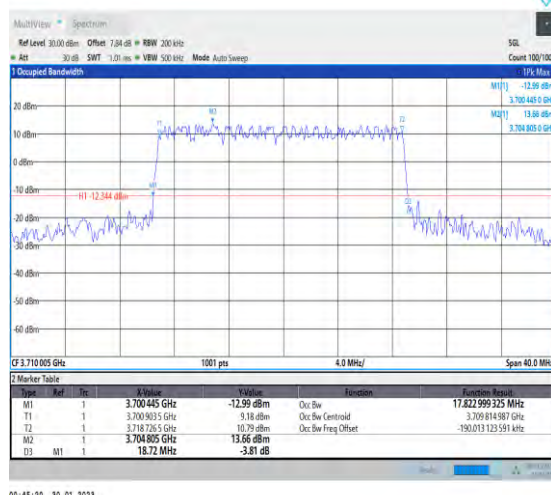
1-N78-3700-3800-30-20-L-4-DFT-64QAM-Outer_Full -50@0-Ant1-17.823-18.720-≤20-PASS
