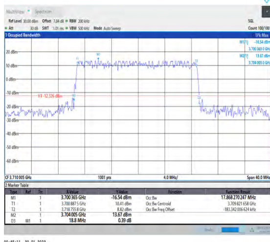
1-N78-3700-3800-30-20-L-3-DFT-16QAM-Outer_Full -50@0-Ant1-17.868-18.800-≤20-PASS
