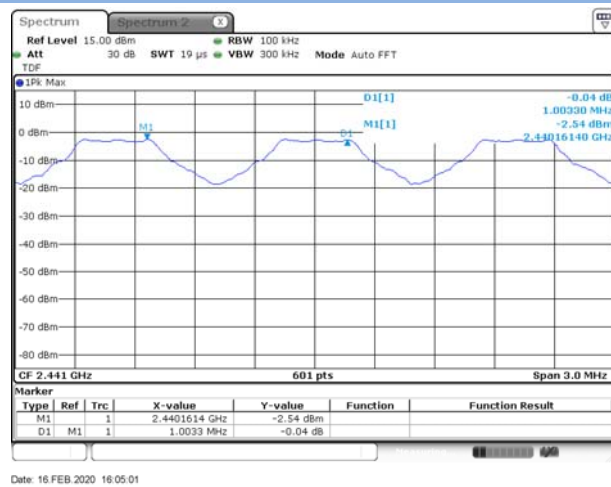
GFSK
