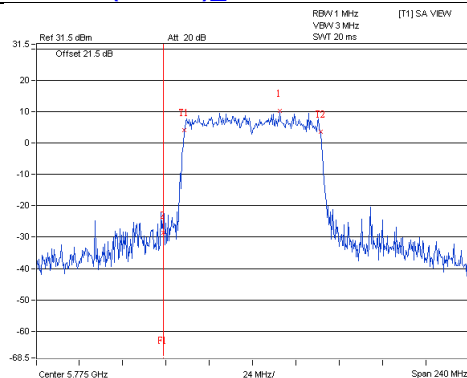
802.11ac(VHT80)_Chain2 / CH149
