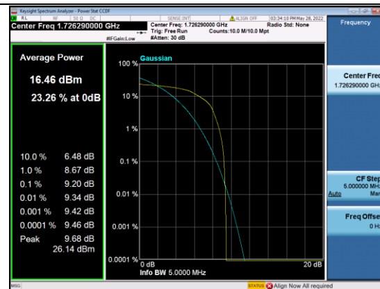
B4-15M-Mid CH-PAPR-Q16
