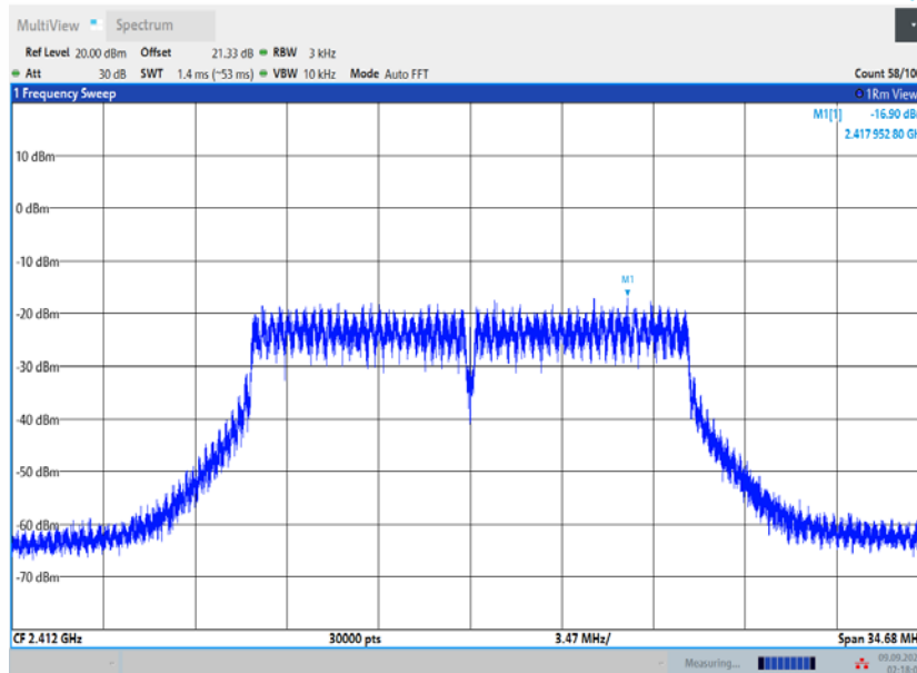
11G_Ant2_2412
