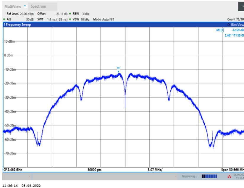
11B_Ant2_2462
