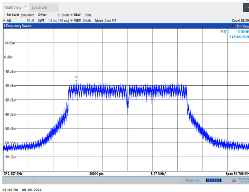
11G_Ant2_2437
