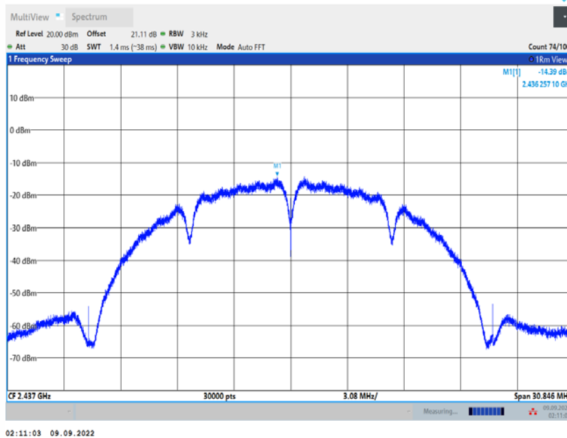
11B_Ant2_2437
