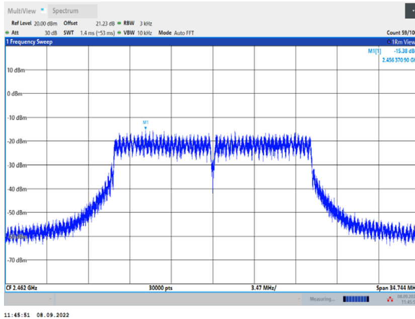
11G_Ant2_2462
