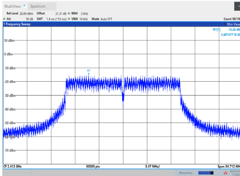
11G_Ant2_2412
