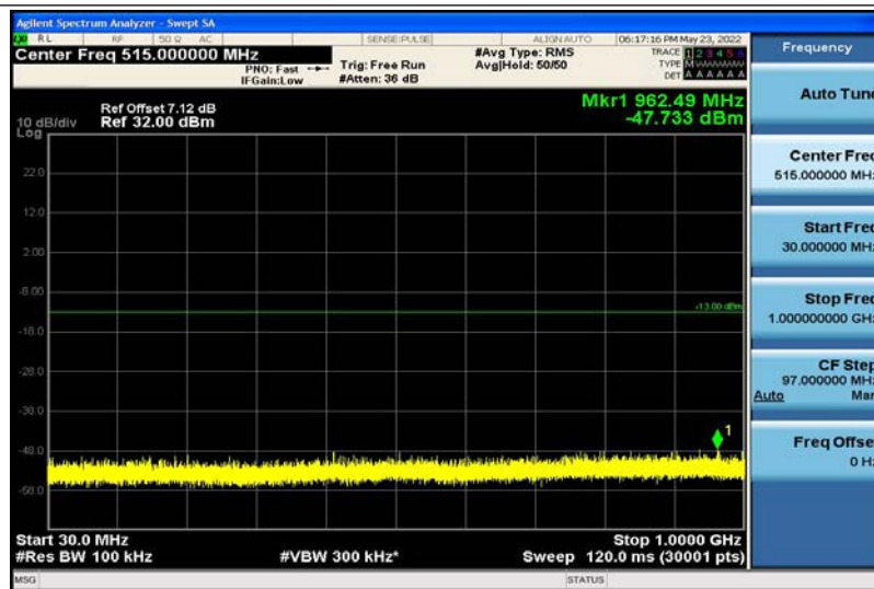
Band2-20MHz-QPSK-18900-1RB#0-30~1000MHz
