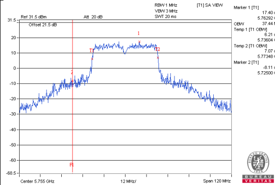
802.11ac(VHT40)_Chain3 / CH151
