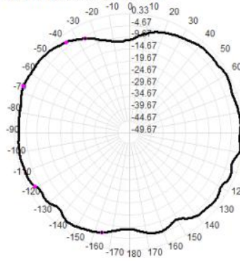
2400.0MHz Total(E2), Max= 0.29dBi
