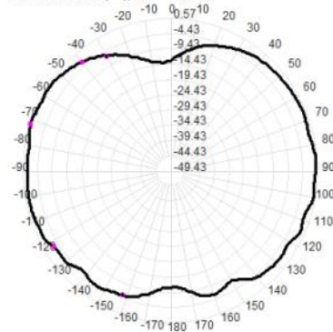
2480.0MHz Total(E2), Max= 0.29dBi
