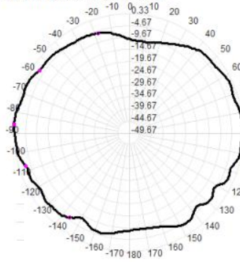
2400.0MHz Total(E1), Max= 0.33dBi
