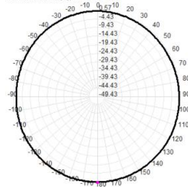
2480.0MHz Total(H), Max= 0.34dBi
