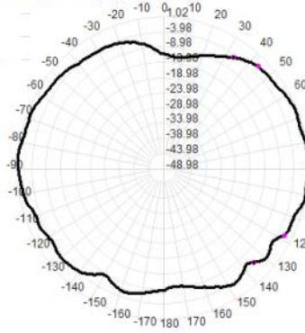
2440.0MHz Total(E1), Max= 0.89dBi
