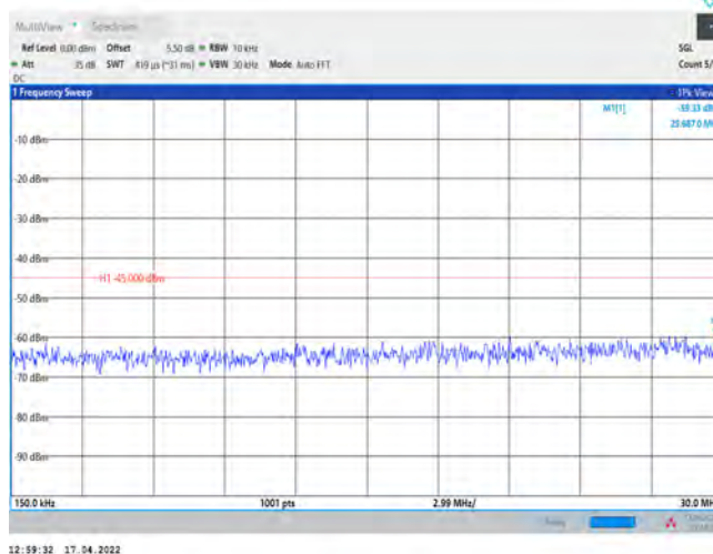
Band38-20MHz-QPSK-37850-1RB#0-Range2:0.15~30MHz
