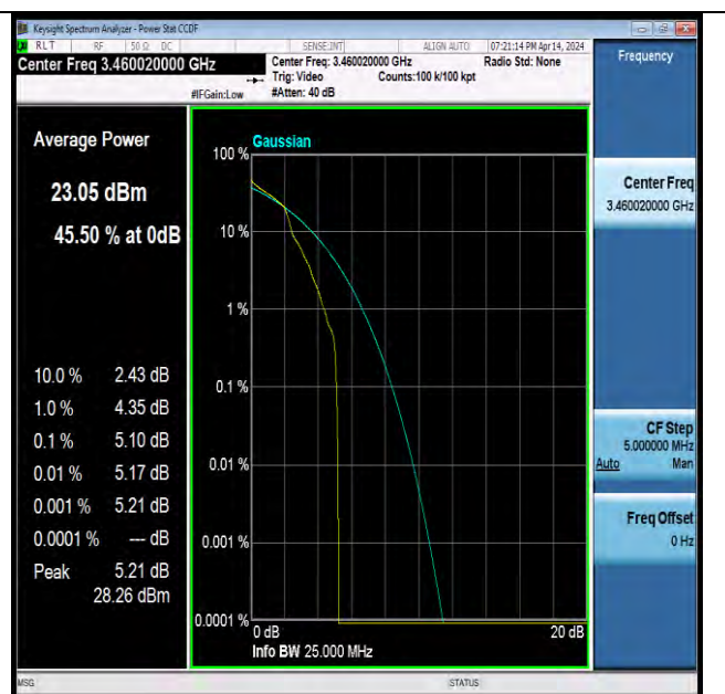
NTNV-N78-3450-3550-PC2-30-20-L-DFT-QPSK-Edge_1RB_Left-PASS
