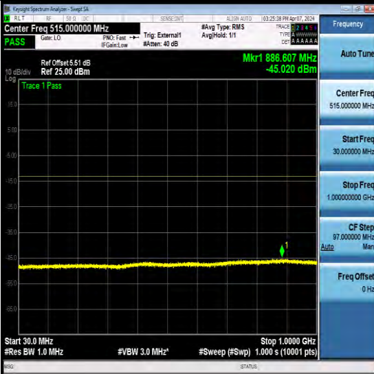
NTNV-N77-3700-3980-PC2-30-60-L-CP-QPSK-Edge_1RB_L eft-Ant5-PASS
