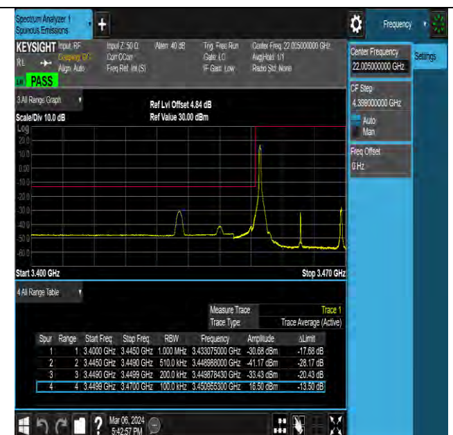
NTNV-N78-3450-3550-PC2-30-20-L-DFT-QPSK-Edge_1RB_Left-Ant5-PASS
