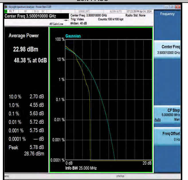
NTNV-N78-3450-3550-PC2-30-20-M-DFT-QPSK-Edge_1RB_Left-PASS
