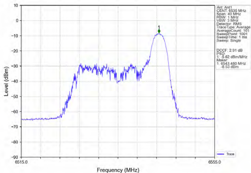
802.11ax(HE20)_LCH_6535MHz_RU26_Right_Ant1_NTNV
