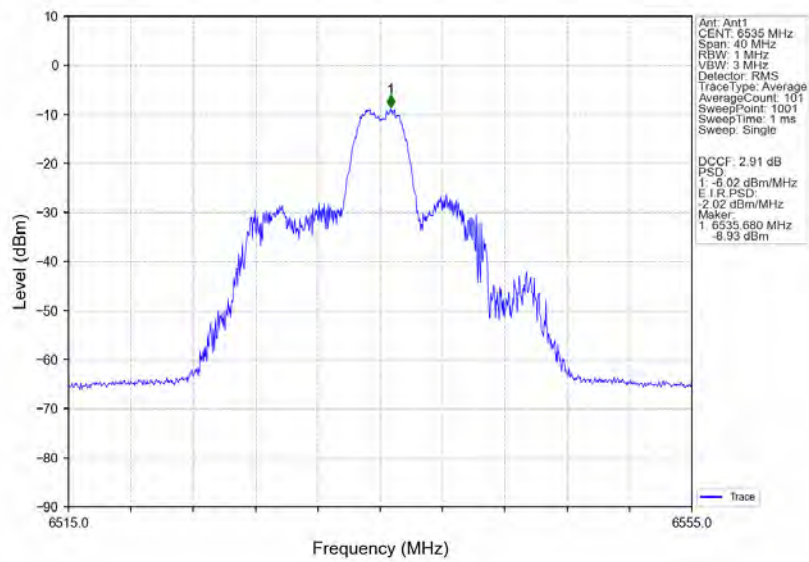
802.11ax(HE20)_LCH_6535MHz_RU26_Right_Ant1_NTNV
