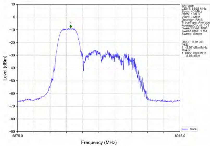
802.11ax(HE20)_LCH_6895MHz_RU52_Right_Ant1_NTNV
