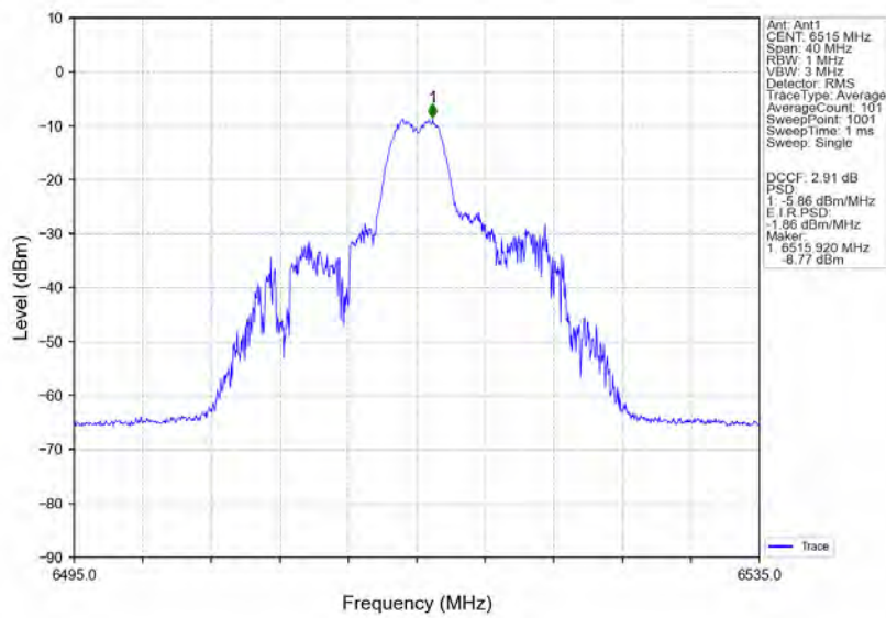
802.11ax(HE20) HCH_6515MHz_RU26_Right_Ant1_NTNV
