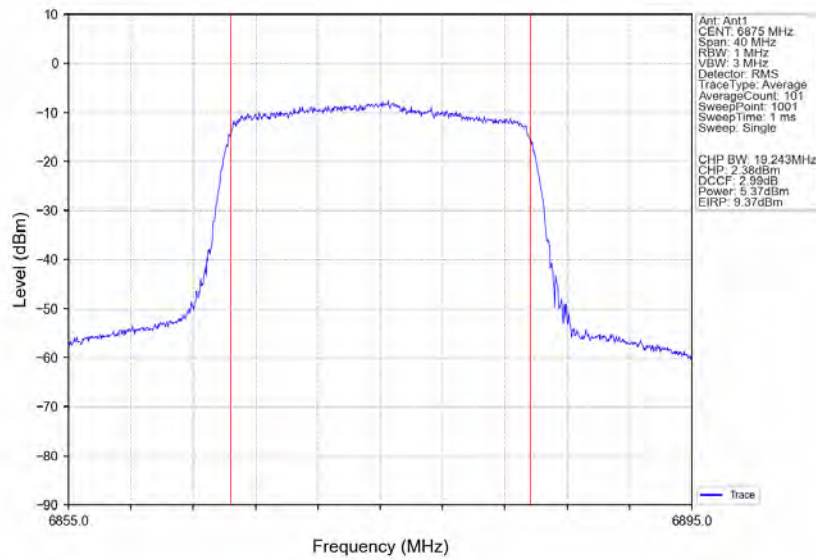
802.11ax(HE20)_HCH_6875MHz_RU242_Ant1_NTNV
