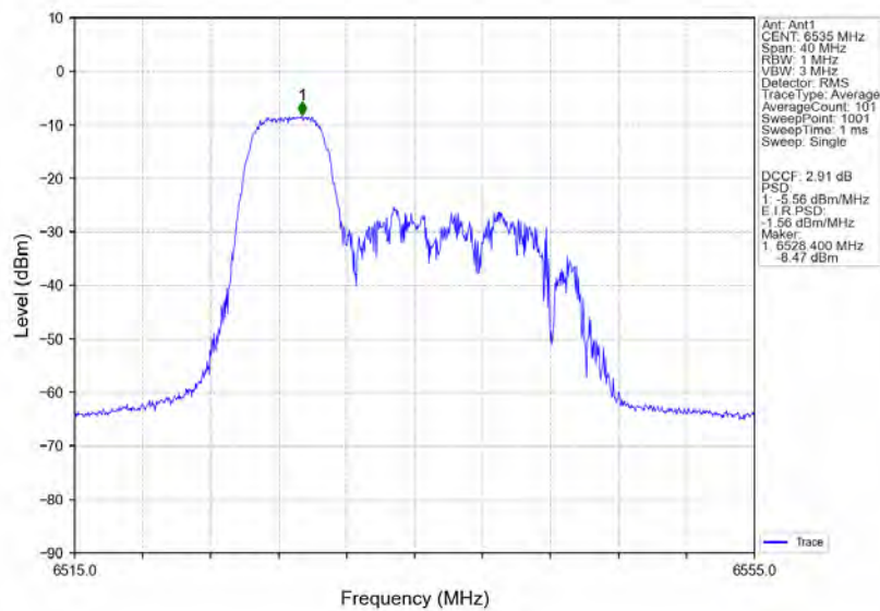
802.11ax(HE20)_LCH_6535MHz_RU52_Right_Ant1_NTNV
