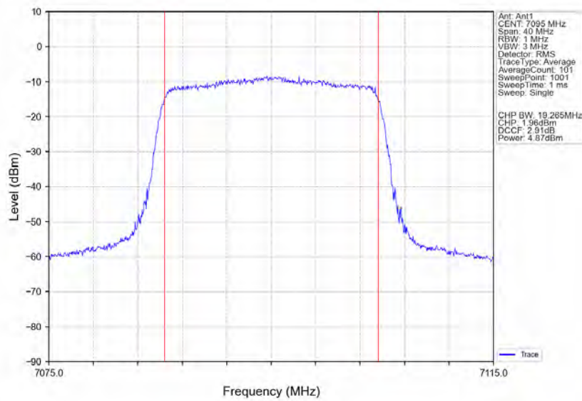
802.11ax(HE20)_HCH_7095MHz_RU242_Ant1_NTNV
