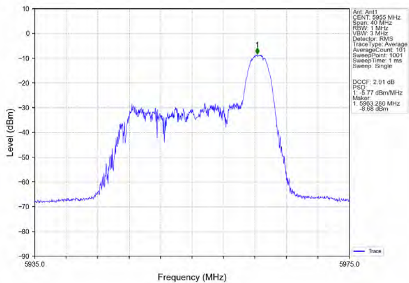
802.11ax(HE20)_LCH_5955MHz_RU26_Right_Ant1_NTNV
