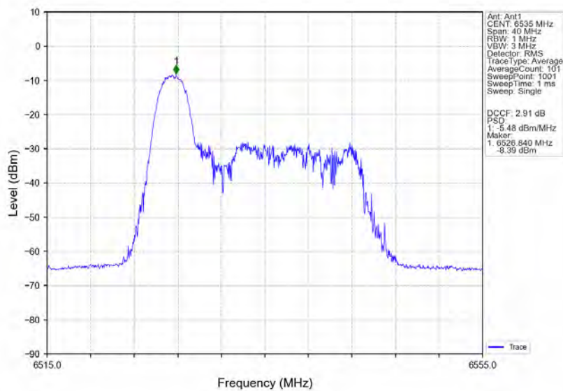
802.11ax(HE20)_LCH_6535MHz_RU26_Left_Ant1_NTNV
