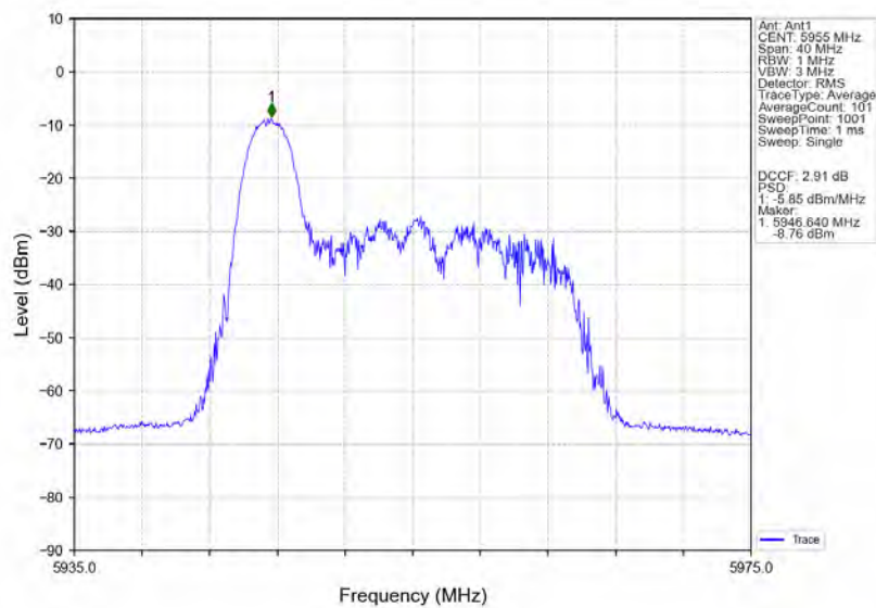
802.11ax(HE20)_LCH_5955MHz_RU26_Left_Ant1_NTNV
