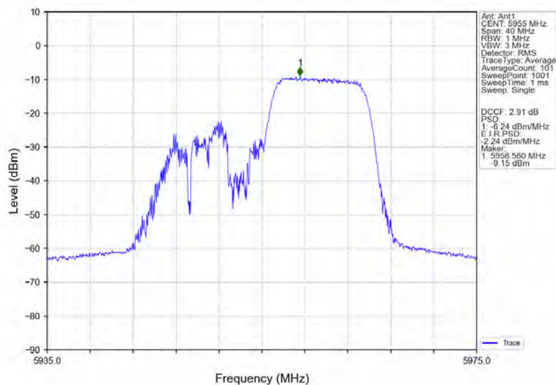
802.11ax(HE20)_LCH_5955MHz_RU106_Right_Ant1_NTNV
