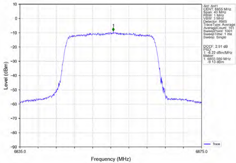
802.11ax(HE20)_HCH_6855MHz_RU242_Ant1_NTNV
