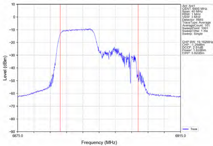
802.11ax(HE20)_LCH_6895MHz_RU106_Right_Ant1_NTNV
