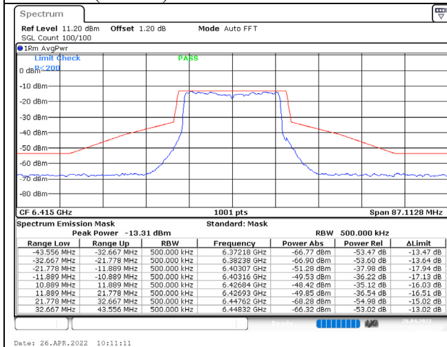
802.11ax (20MHz) / 6415MHz / Chain A / NSS-1
