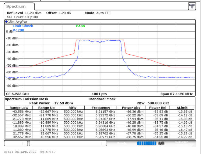
802.11ax (20MHz) / 6255MHz / Chain D / NSS-1
