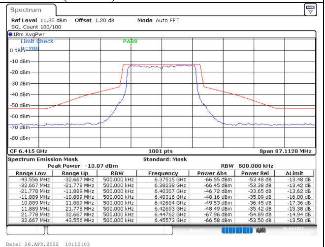
802.11ax (20MHz) / 6415MHz / Chain B / NSS-1
