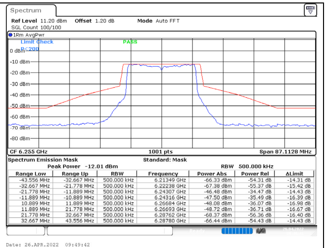
802.11ax (20MHz) / 6255MHz / Chain B / NSS-1
