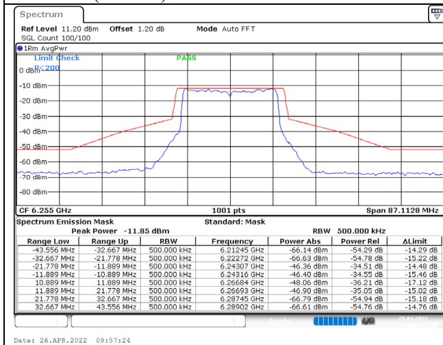
802.11ax (20MHz) / 6255MHz / Chain C / NSS-1
