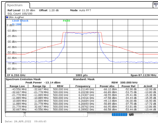
802.11ax (20MHz) / 6255MHz / Chain A / NSS-1
