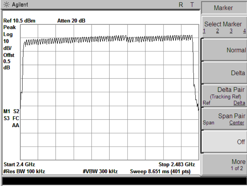
8DPSK Mode
