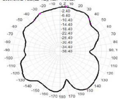
2500.0MHz Total(E2-YZ), Max= 1.60dBi
