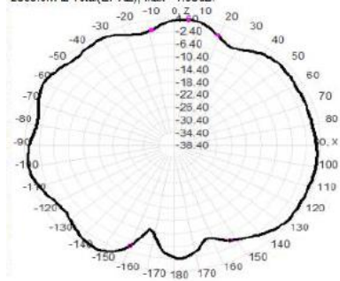
2500.0MHz Total(E1-XZ), Max= 1.55dBi
