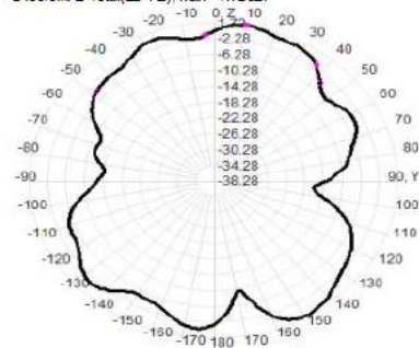
2450.0MHz Total(E2-YZ), Max= 1.72dBi
