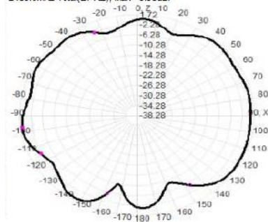
2450.0MHz Total(E1-XZ), Max= 0.95dBi
