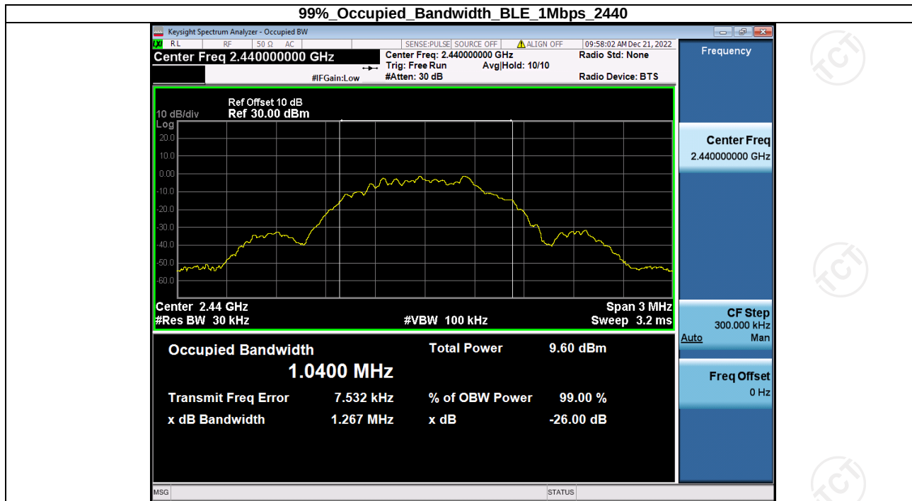
99% Occupied Bandwidth BLE 1Mbps 2440
