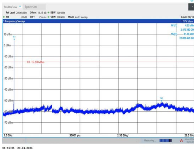
BLE_1M_Ant1_2480_1000~26500
