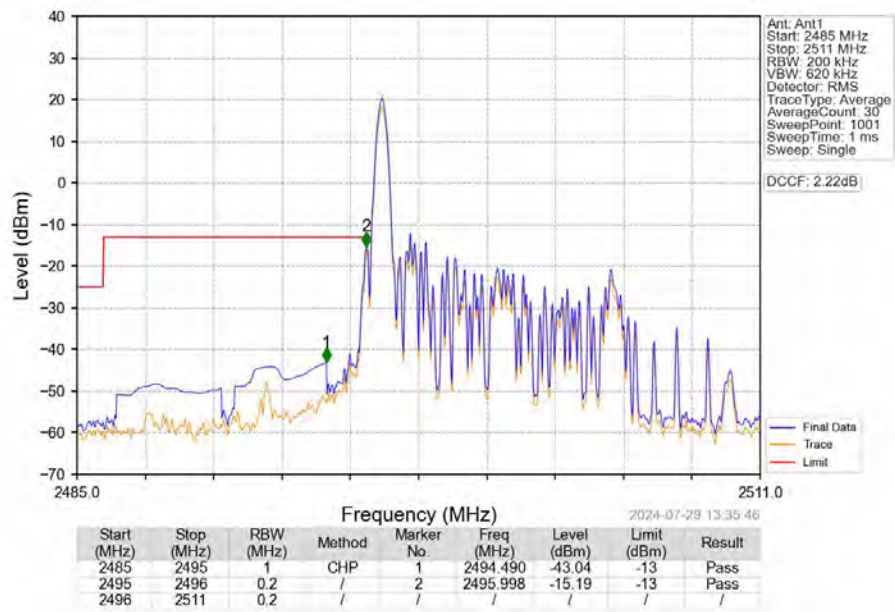
Band41_10MHz_16QAM_LCH_2501MHz_RB_1_0_NTNV
