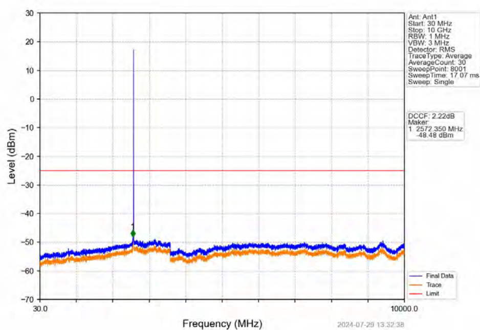
Band41_5MHz_QPSK_MCH_2593MHz_RB_1_0_NTNV
