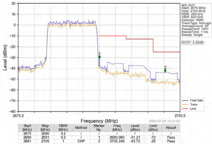
Band41_10MHz_QPSK_HCH_2685MHz_RB_50_0_NTNV
