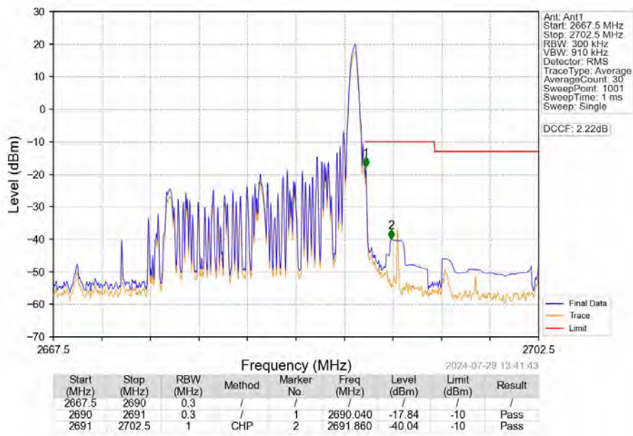
Band41_15MHz_QPSK_HCH_2682.5MHz_RB_1_74_NTNV
