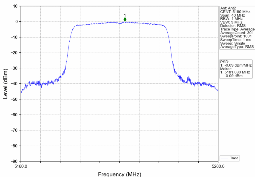
802.11ax(HEW20)_LCH_5180MHz_RU242_Left_Ant2_NTNV
