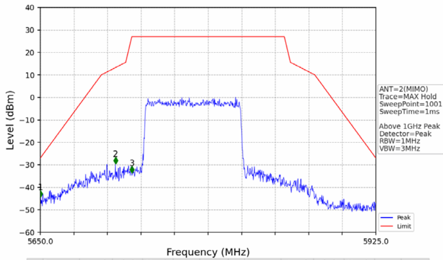
802.11ax(HEW80)_MCH_5775MHz_RU996_Left_Ant2_NTNV
