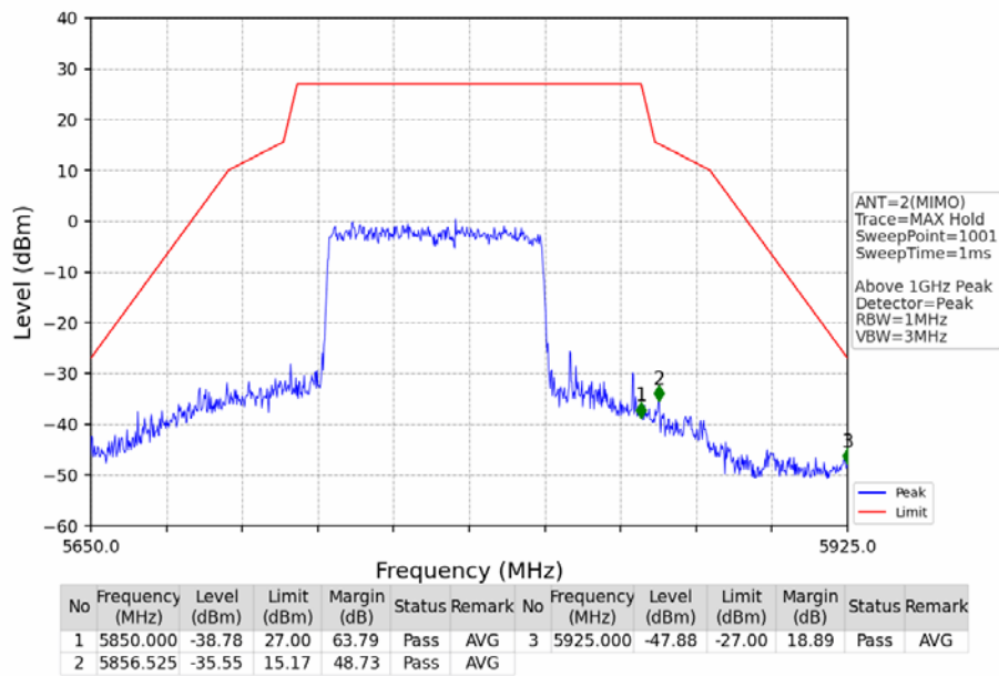
802.11ax(HEW80)_MCH_5775MHz_RU996_Left_Ant2_NTNV
