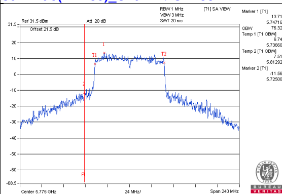
802.11ac(VHT80)_Chain1 / CH155
