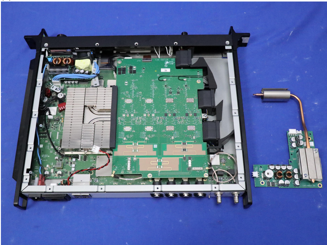
(9) EUT Photo
