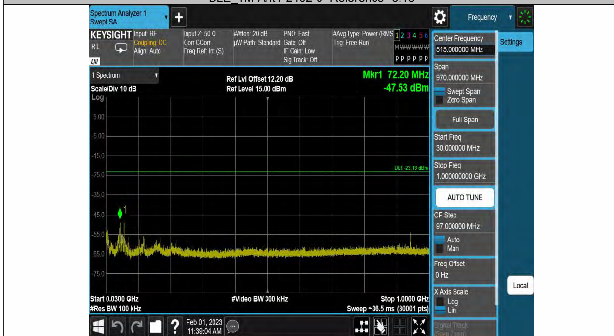
BLE_1M-Ant1-2402-30~1000--3.18
