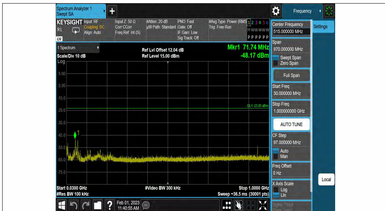
BLE_1M-Ant1-2440-30~1000--3.05
