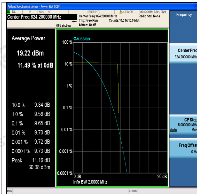
GSM850-128-PASS
