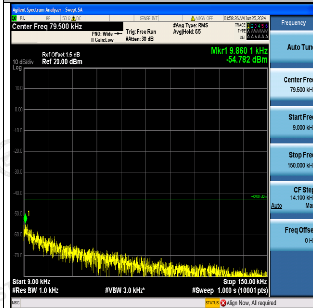
GSM1900-810-0-0.009-0.15MHz-PASS
