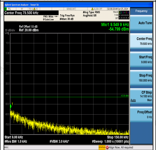
GPRS1900-810-0-0.009-0.15MHz-PASS
