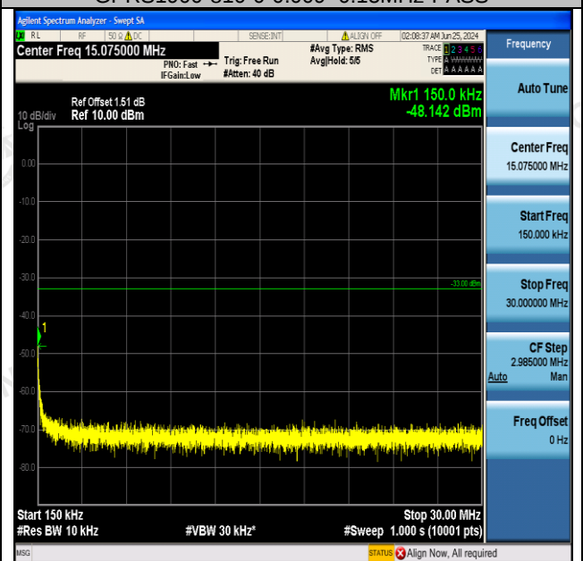
GPRS1900-810-0-0.15-30MHz-PASS
