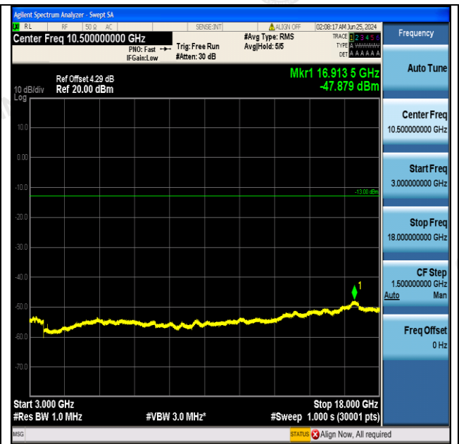
GPRS1900-661-0-3000-18000MHz-PASS
