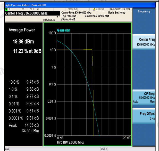
GPRS850-190-PASS
