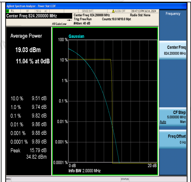
GPRS850-128-PASS
