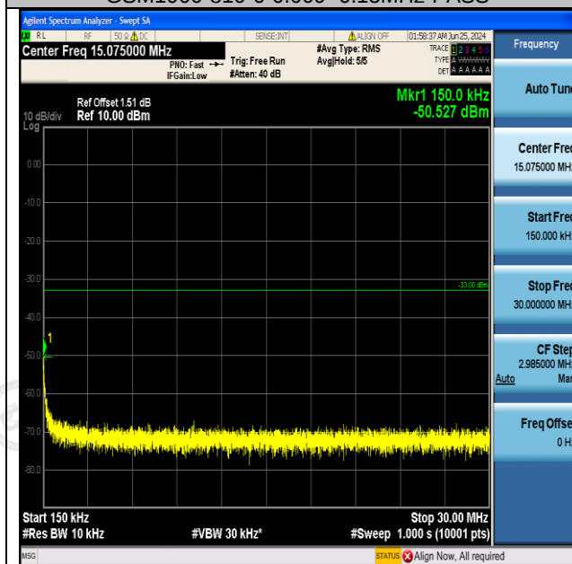
GSM1900-810-0-0.15-30MHz-PASS
