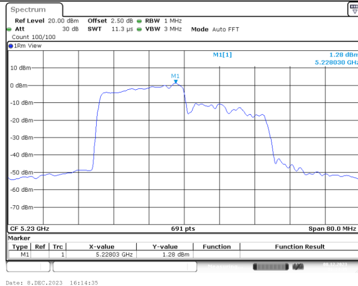
11AX40MIMO_Ant4_5230_242Tone_RU61
