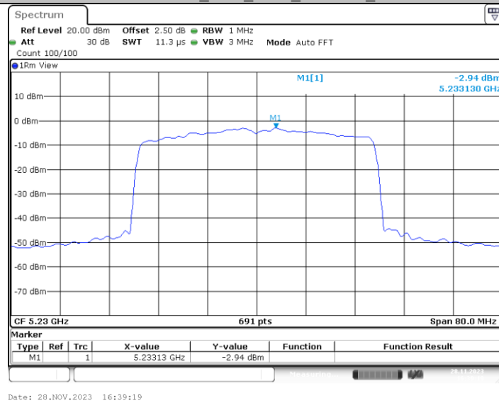
11AX40MIMO_Ant1_5230_484Tone_RU65
