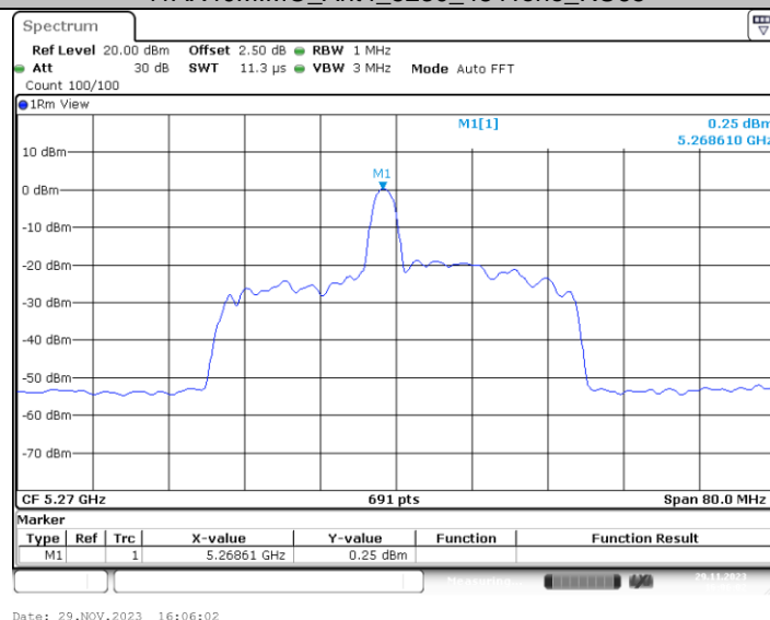
11AX40MIMO_Ant1_5270_26Tone_RU8
