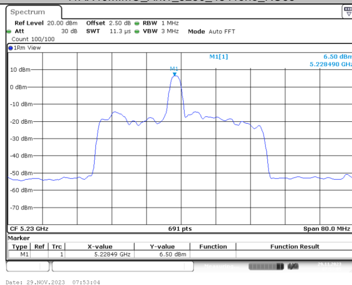
11AX40MIMO_Ant2_5230_26Tone_RU8
