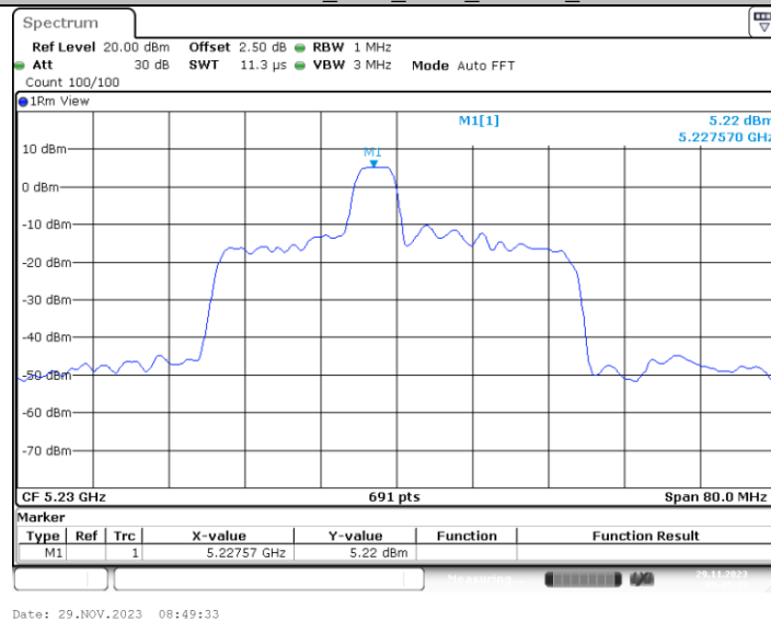
11AX40MIMO_Ant4_5230_52Tone_RU40
