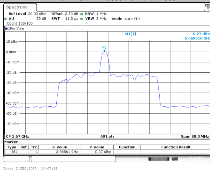
11AX40MIMO_Ant1_5670_26Tone_RU8
