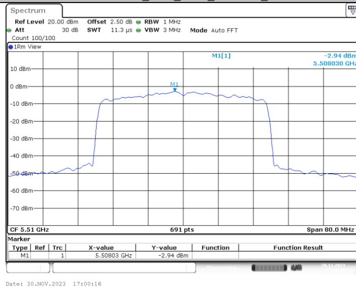
11AX40MIMO_Ant1_5510_484Tone_RU65
