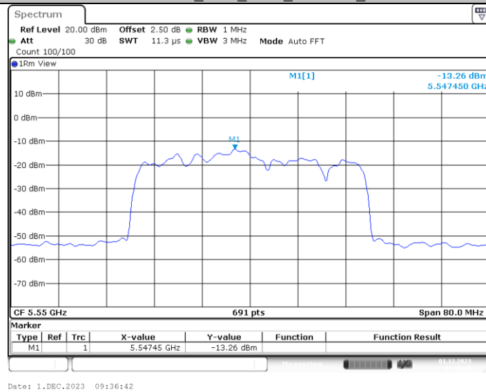
11AX40MIMO_Ant4_5550_484Tone_RU65
