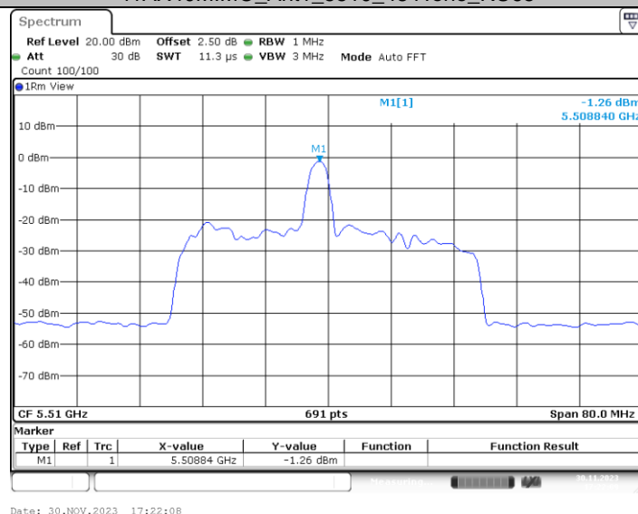
11AX40MIMO_Ant2_5510_26Tone_RU8
