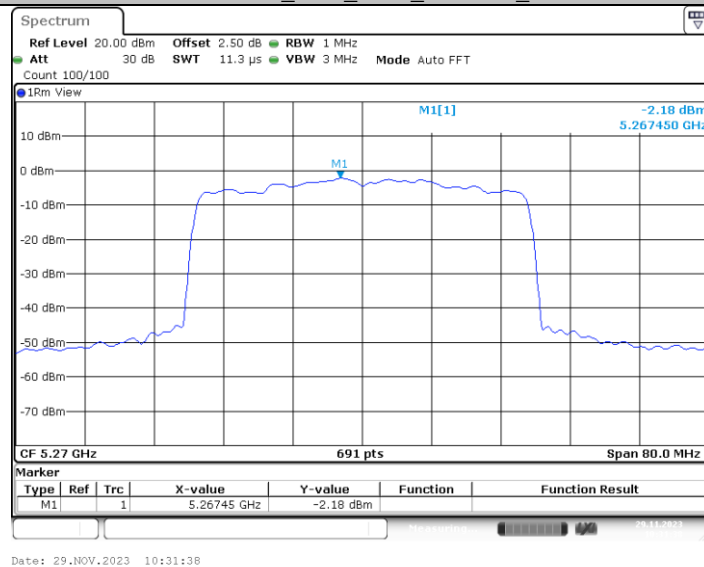
11AX40MIMO_Ant3_5270_484Tone_RU65
