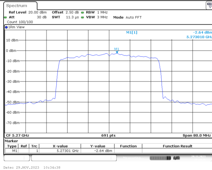
11AX40MIMO_Ant4_5270_484Tone_RU65
