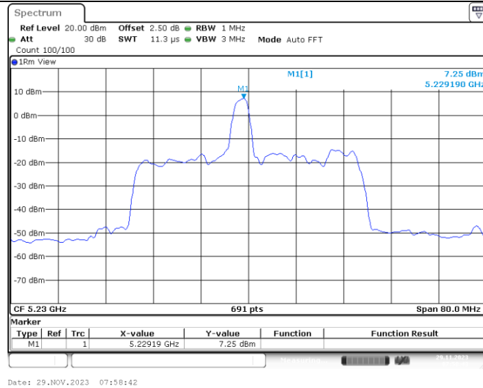
11AX40MIMO_Ant4_5230_26Tone_RU8
