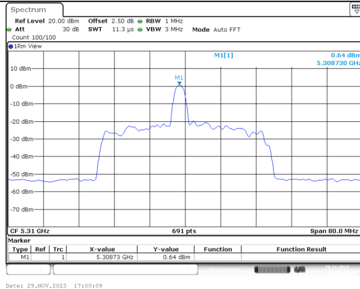
11AX40MIMO_Ant1_5310_26Tone_RU8
