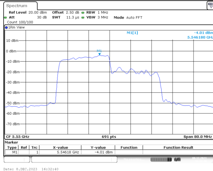
11AX40MIMO_Ant1_5550_242Tone_RU61
