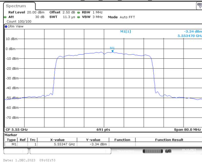
11AX40MIMO_Ant1_5550_484Tone_RU65
