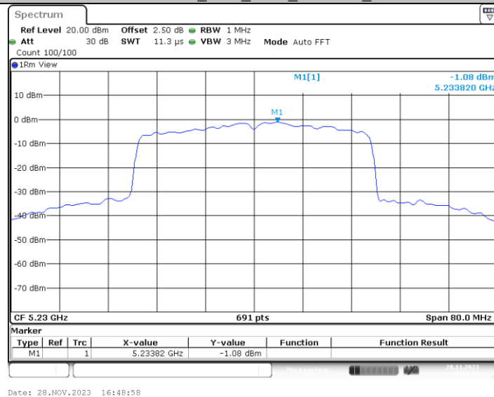
11AX40MIMO_Ant4_5230_484Tone_RU65
