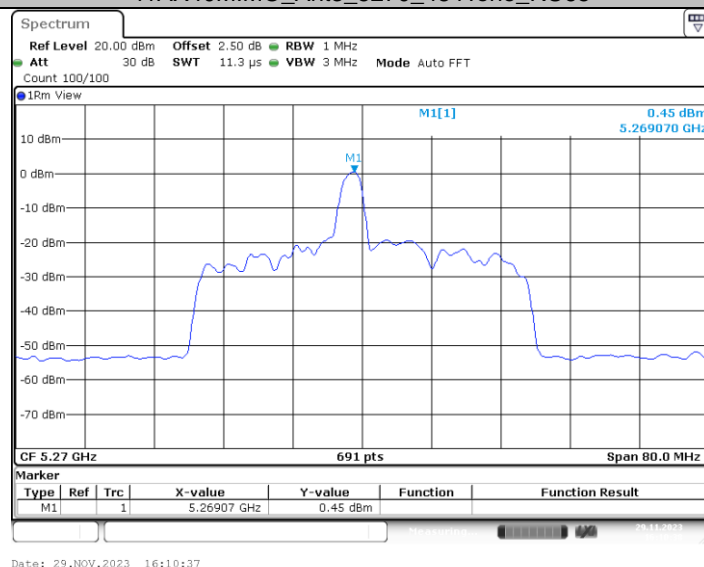
11AX40MIMO_Ant4_5270_26Tone_RU8
