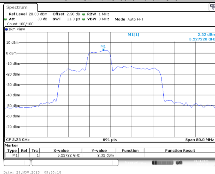
11AX40MIMO_Ant4_5230_106Tone_RU54
