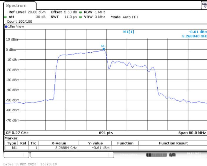
11AX40MIMO_Ant3_5270_242Tone_RU61
