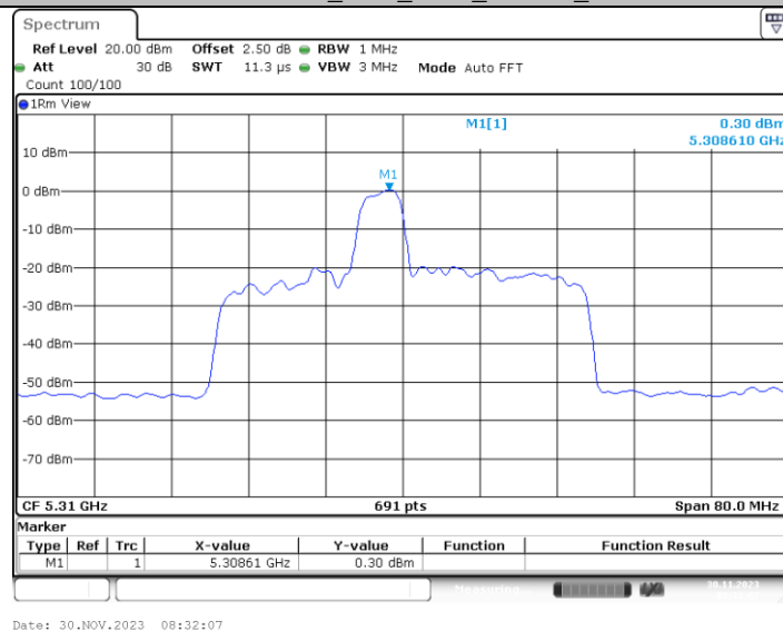
11AX40MIMO_Ant1_5310_52Tone_RU40
