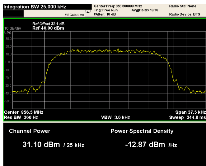
Mod. iDEN
