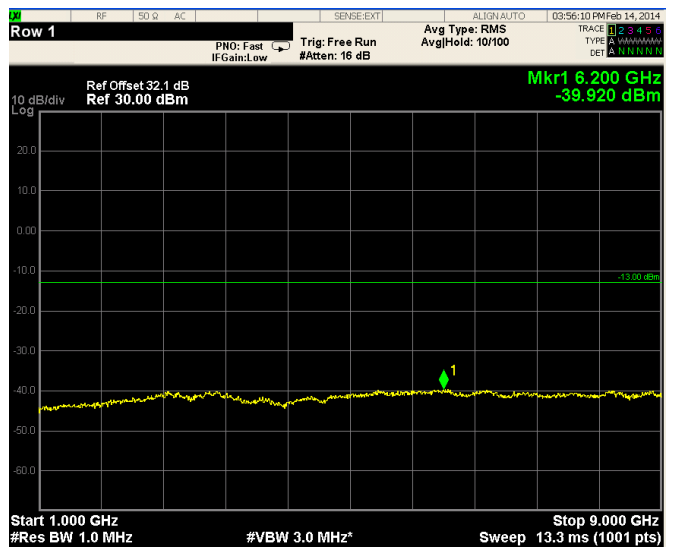
1GHz-9GHz
