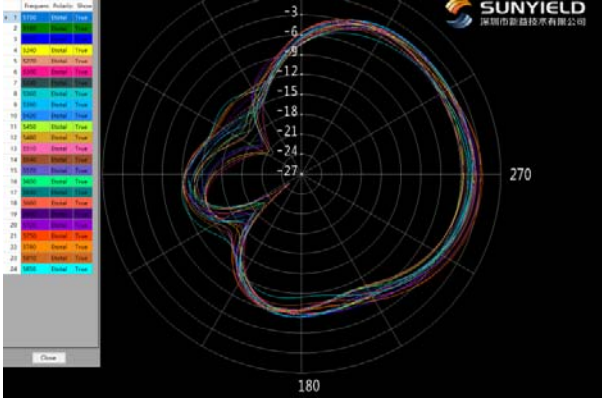
5G WIFI Theta=90deg
