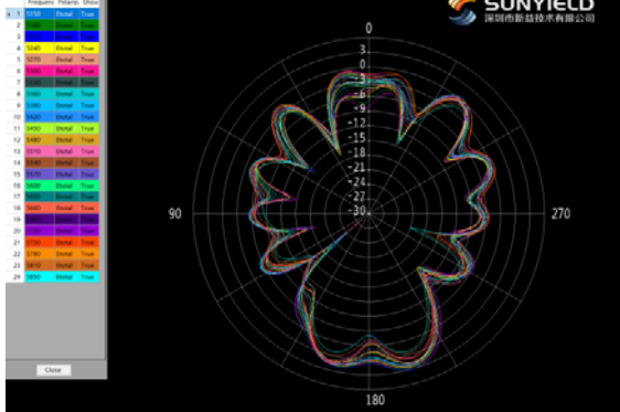
5G WIFI Phi=0deg
