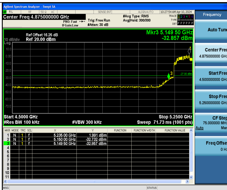
11AC80SISO-Ant2-5210-PASS
