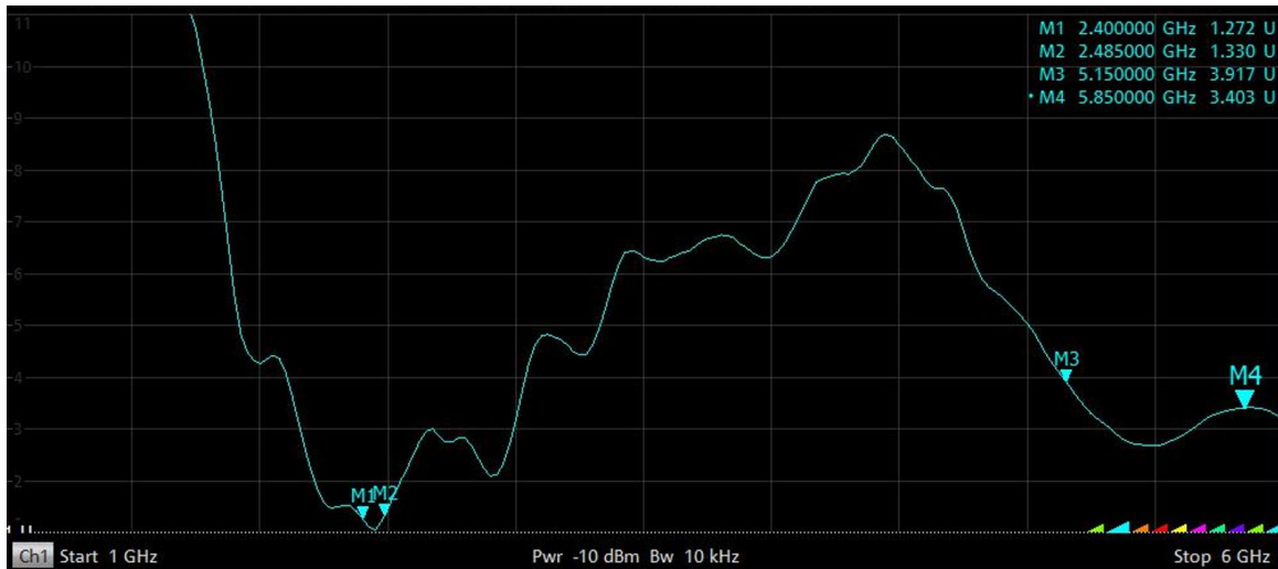
BT/WIFI Antenna
