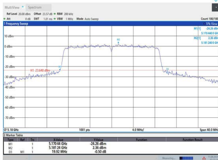
11AC20MIMO_Ant2_5180
