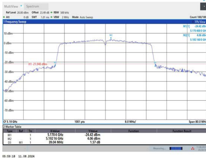
11AC40MIMO_Ant2_5190
