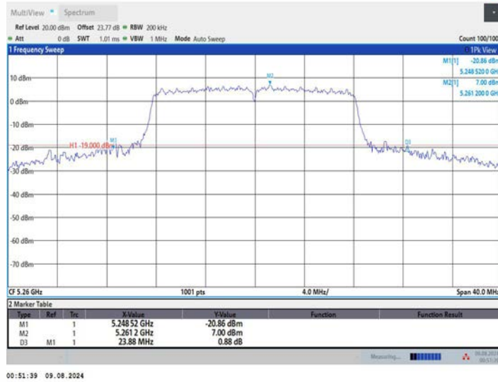
11A_Ant3_5260
