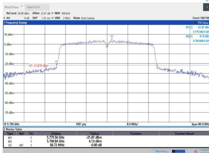
11N40MIMO_Ant3_5795
