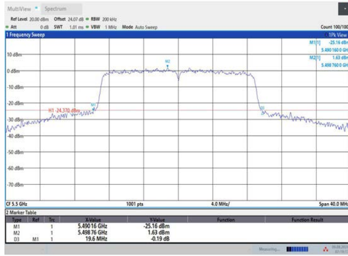
11N20MIMO_Ant2_5500
