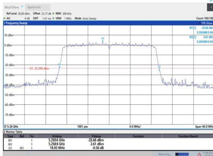
11AC20MIMO_Ant3_5260
