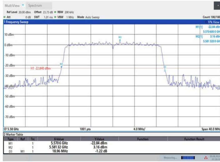
11N20MIMO_Ant3_5580
