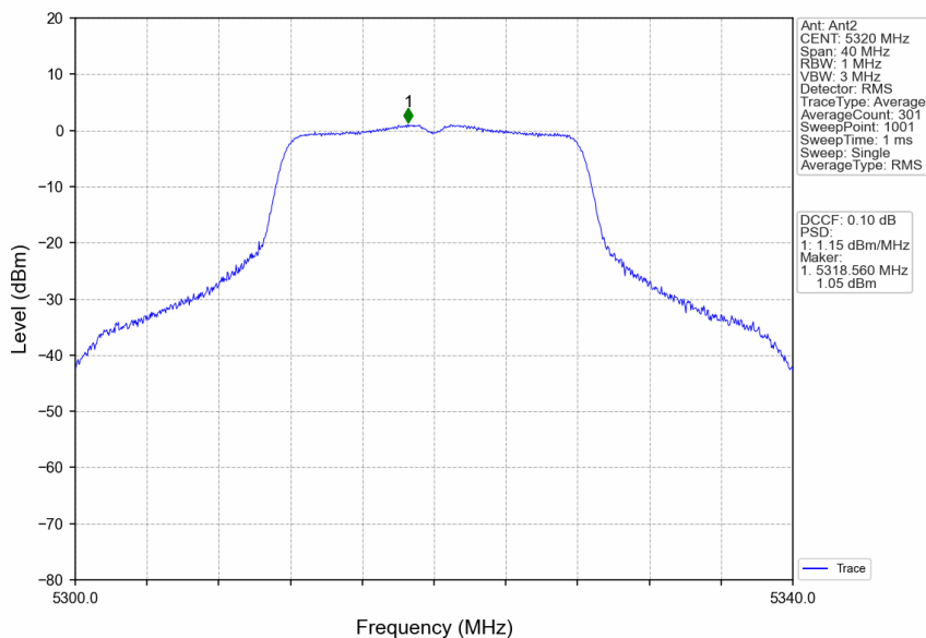
802.11a_HCH_5320MHz_MIMO_NTNV
