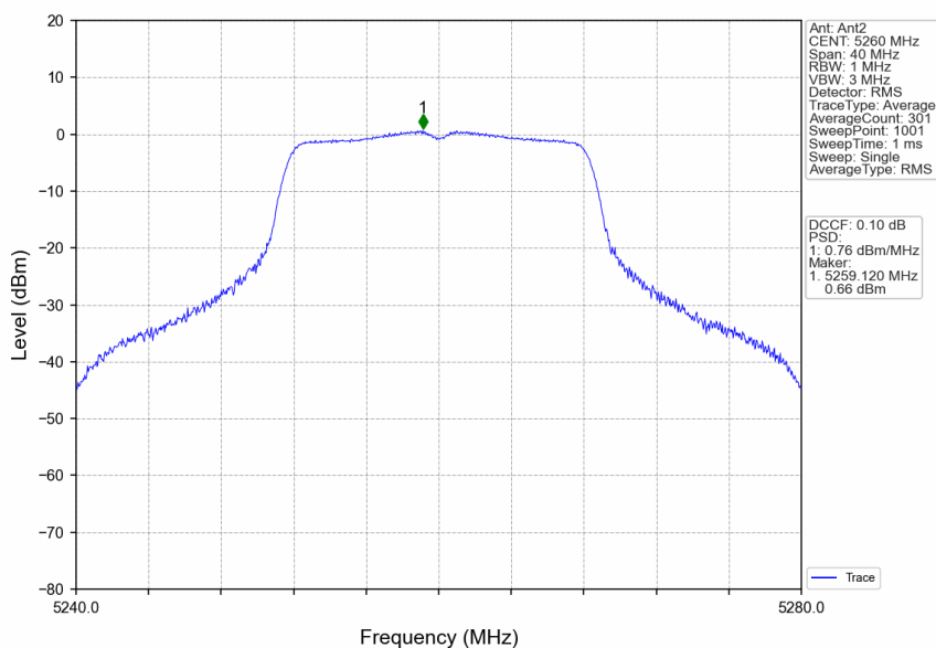
802.11a_LCH_5260MHz_MIMO_NTNV
