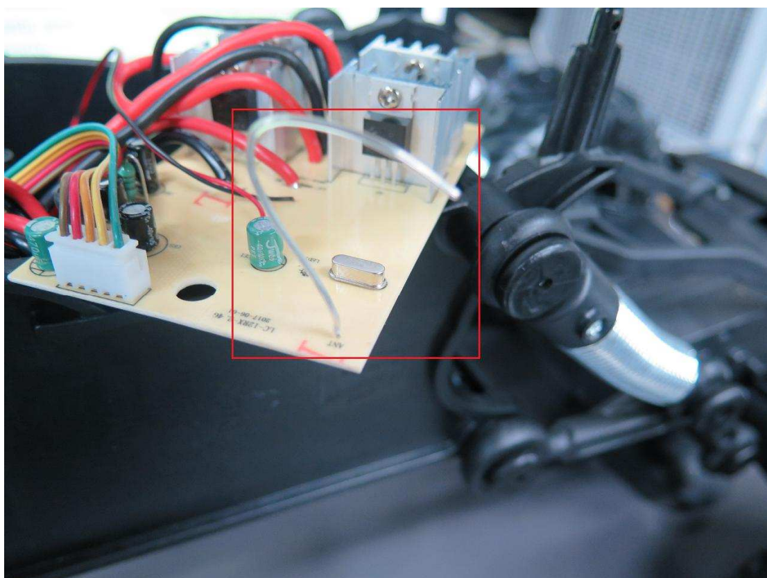
EUT antenna
