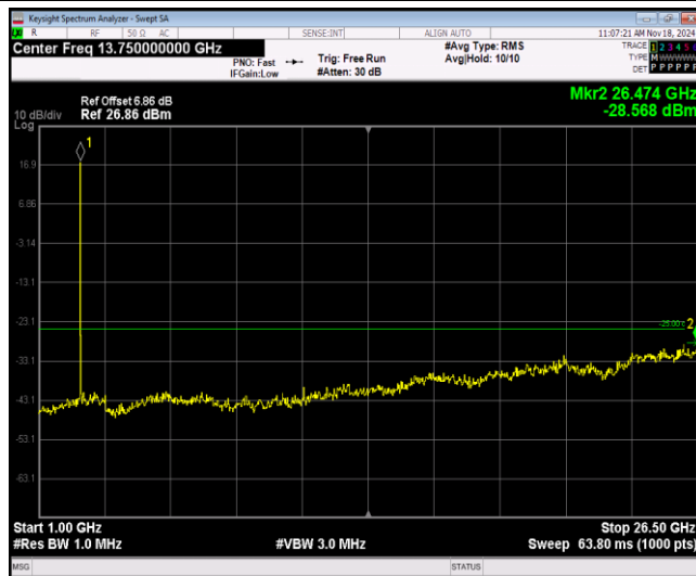
Band38-20MHz-QPSK-37850-1RB#0-Range2:1000~26500MHz
