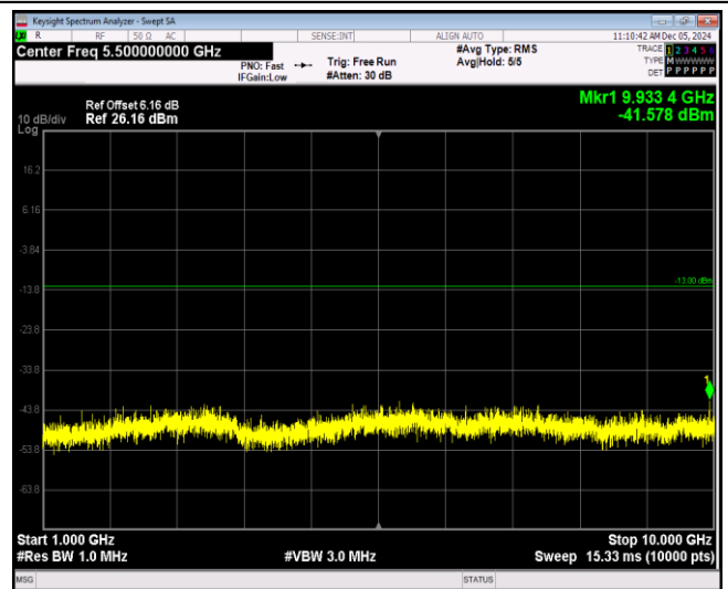
Band5-10MHz-QPSK-20600-1RB#0-Range2:1000~1 0000MHz
