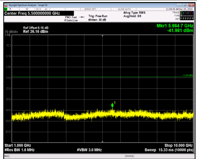
Band5-10MHz-QPSK-20525-1RB#0-Range2:1000~1 0000MHz
