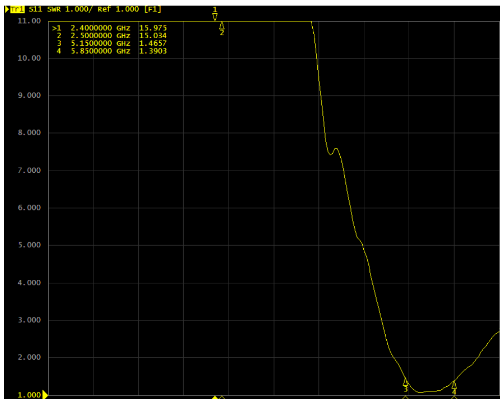
VSWR-3
