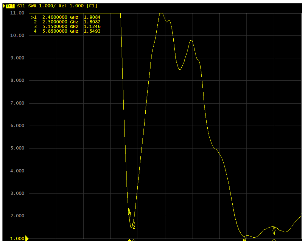
VSWR-1
