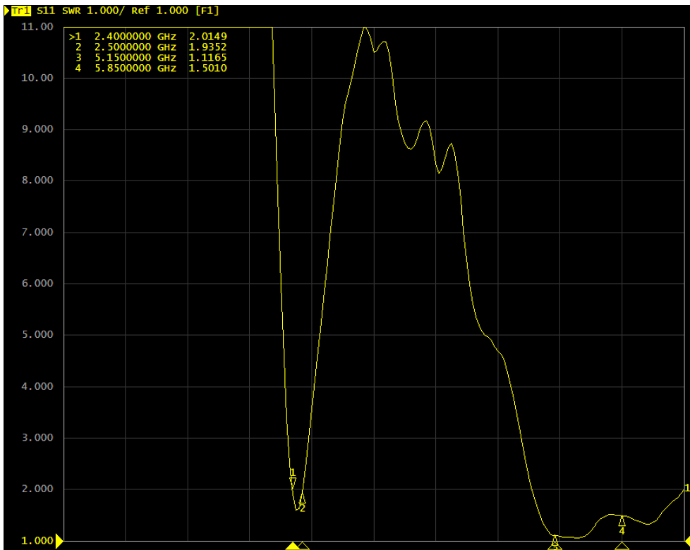
VSWR-2
