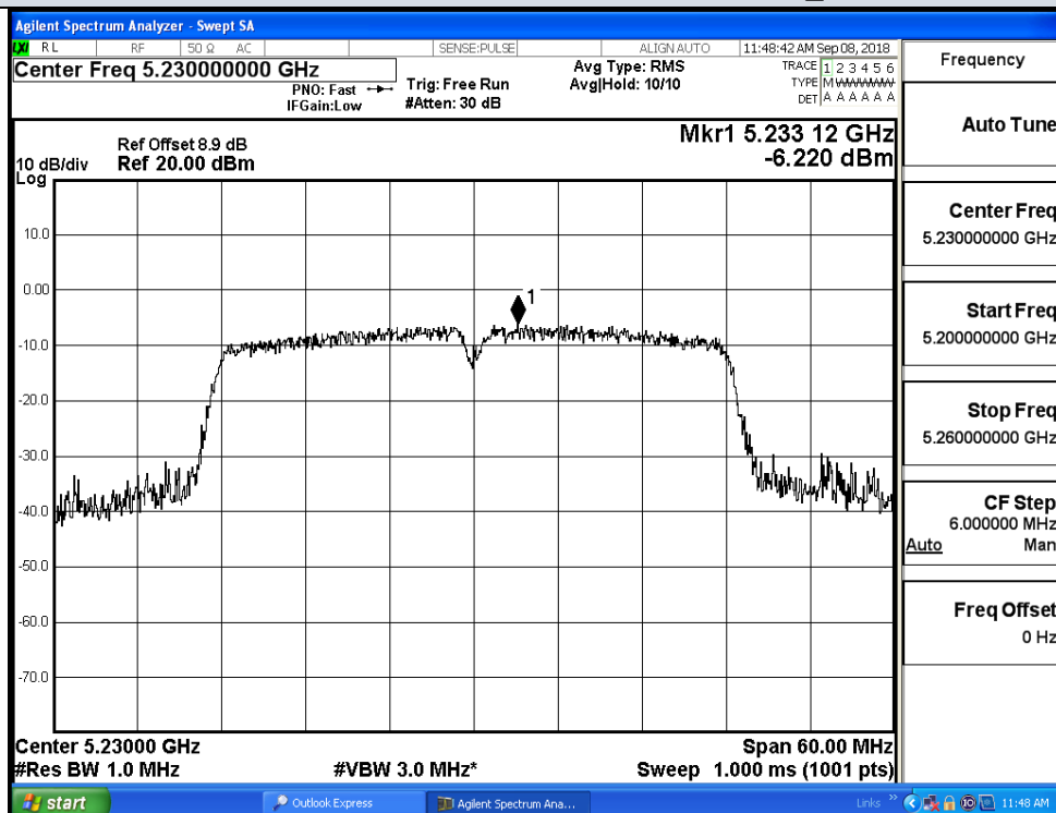
IEEE 802.11n HT40 / Channel 46 / 5230 MHz_Ant0
