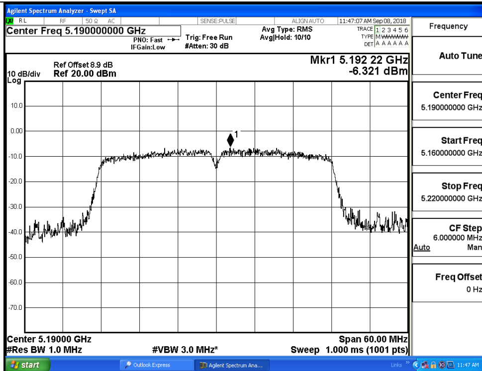
IEEE 802.11n HT40 / Channel 38 / 5190 MHz_Ant0
