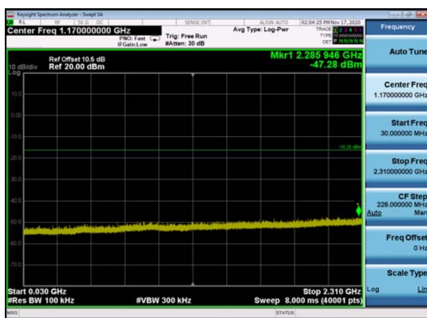
,Plot 3,30MHz~2310MHz-802.11g,2437MHz
