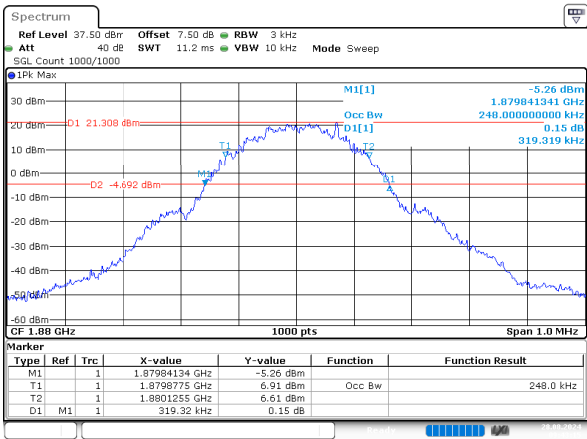
GSM_Middle 0.248MHz
