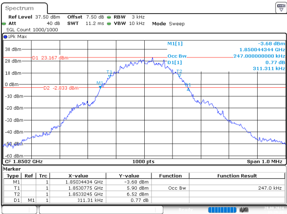
GSM_Low 0.247MHz
