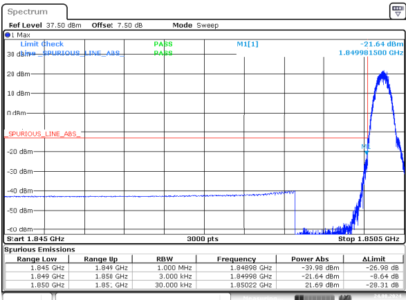
GSM_Low -21.64dBm
