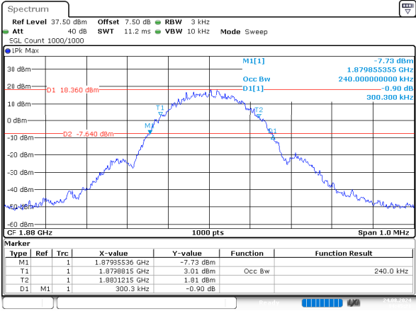
EDGE_Middle_Solt1 0.240MHz
