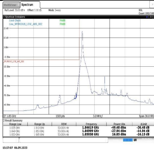
Band2-10MHz-QPSK-18650-50RB#0
