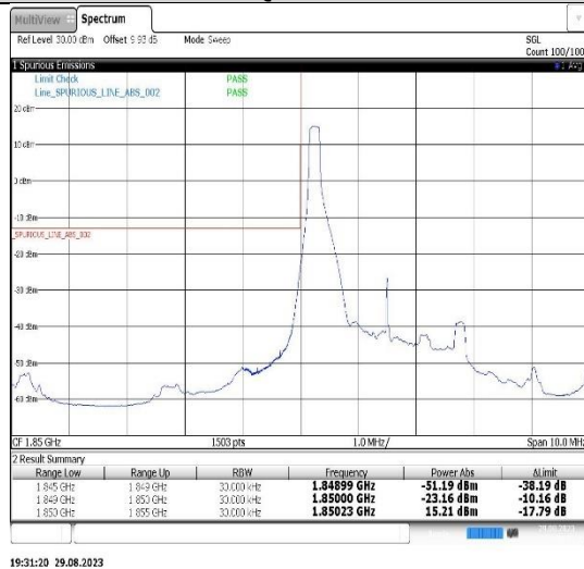
Band2-3MHz-QPSK-18615-1RB#0
