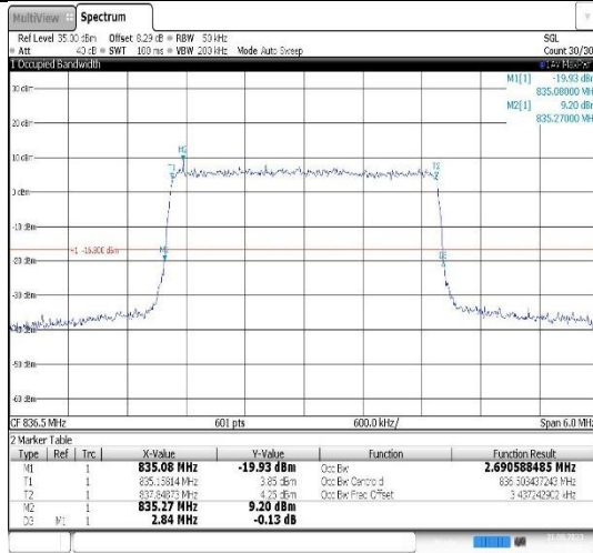
Band26(824-849)-3MHz-QPSK-26915-15RB#0
