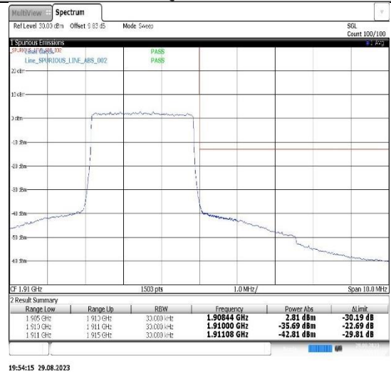
Band2-3MHz-16QAM-18615-15RB#0
