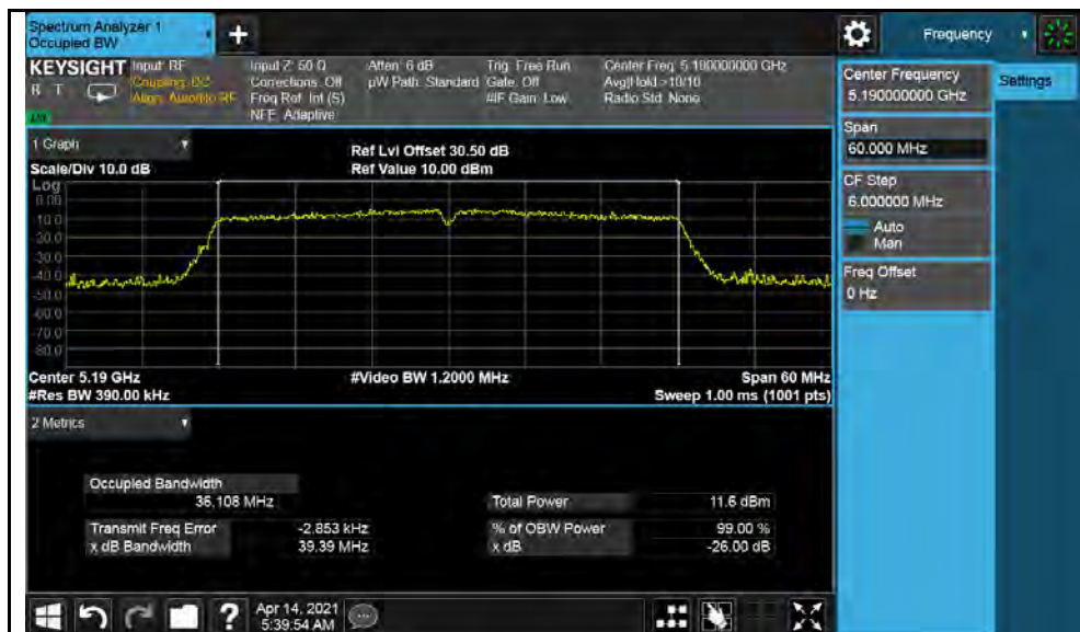
802.11n-HT40-5190MHz
