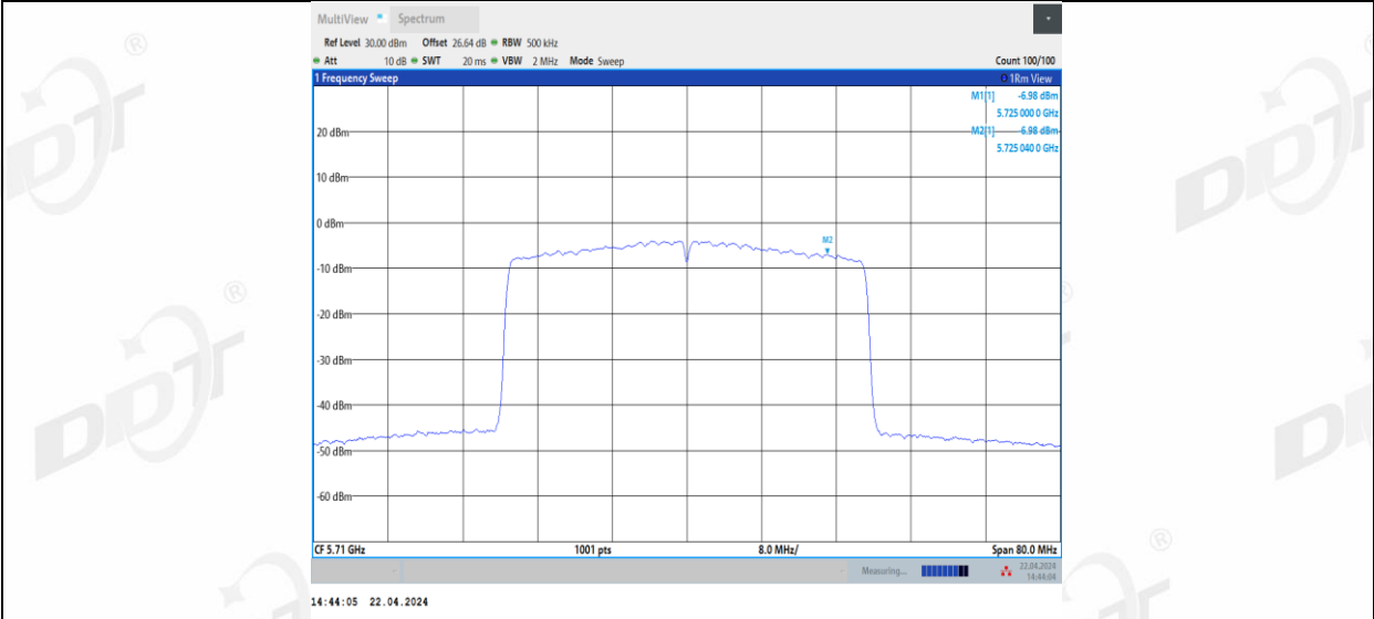
11AX40MIMO_Ant3_5710_UNII-3
