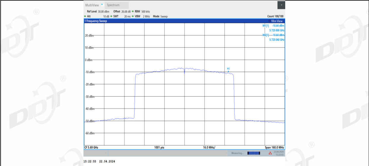
11AX80MIMO_Ant3_5690_UNII-3
