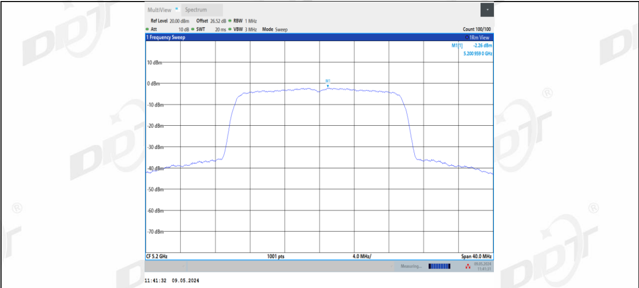
11BE20MIMO Ant2_5200
