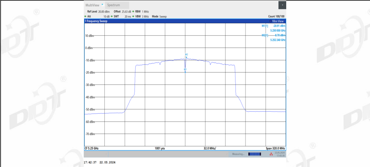
11AX160MIMO_Ant3_5250_UNII-2A
