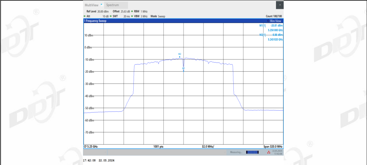
11AX160MIMO_Ant3_5250_UNII-1
