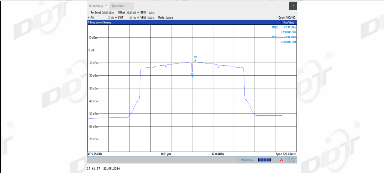
11AX160MIMO_Ant2_5250_UNII-2A
