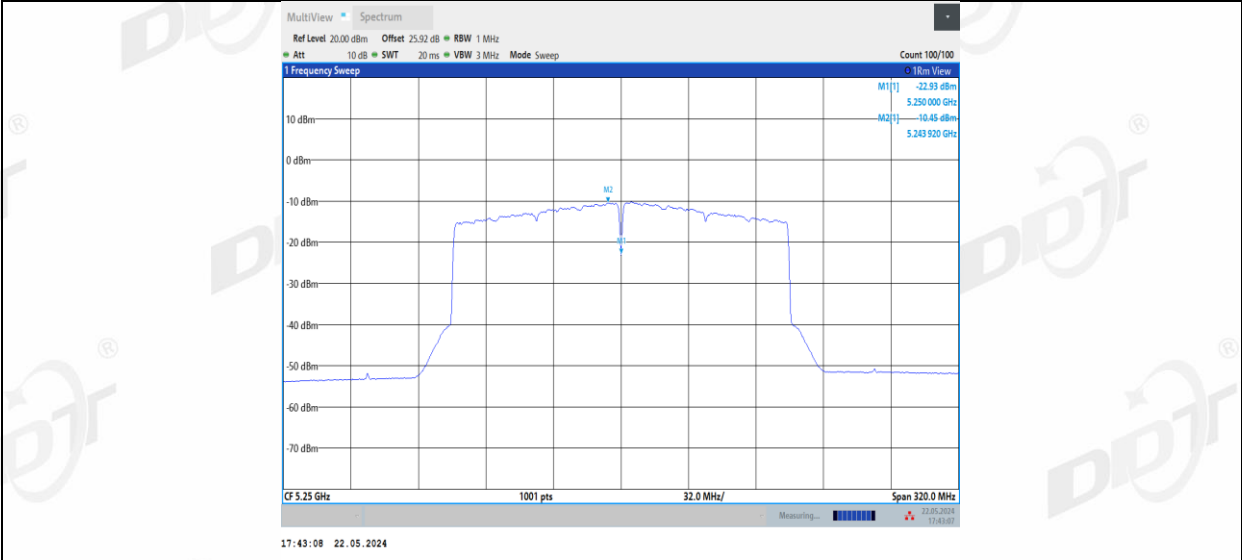
11AX160MIMO_Ant1_5250_UNII-2A
