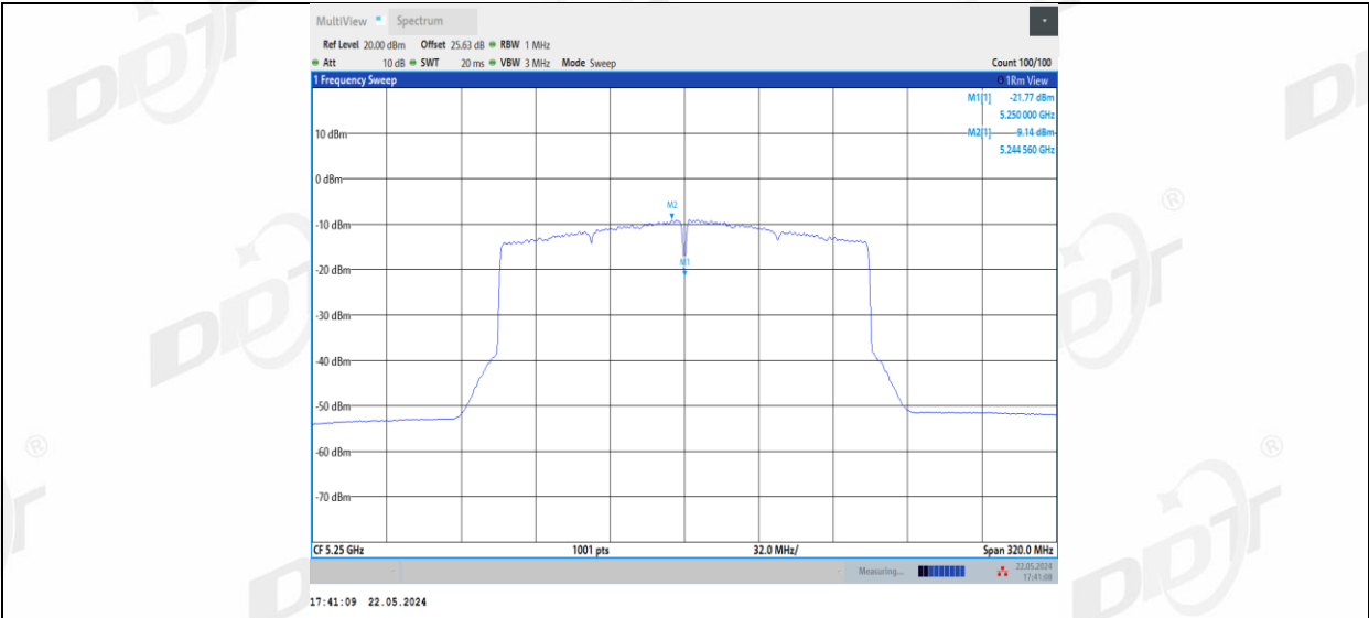
11AX160MIMO_Ant2_5250_UNII-1
