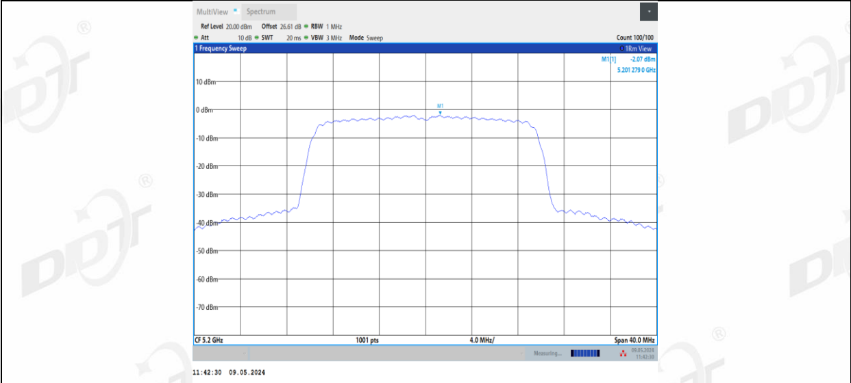
11BE20MIMO Ant3_5200
